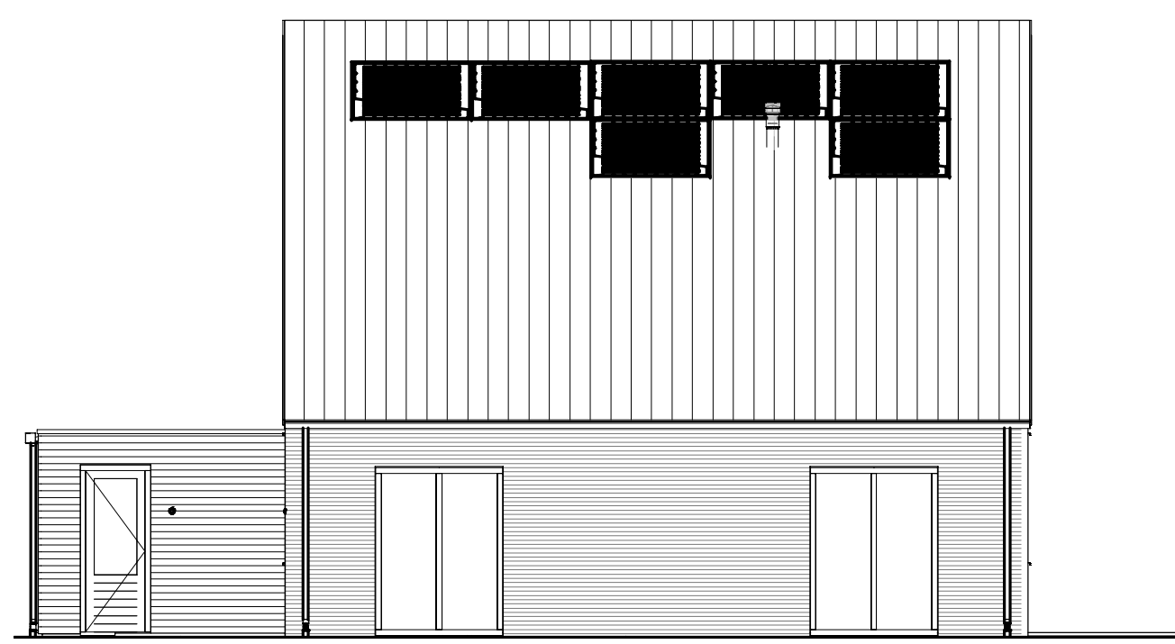
linkergevel 1:100
