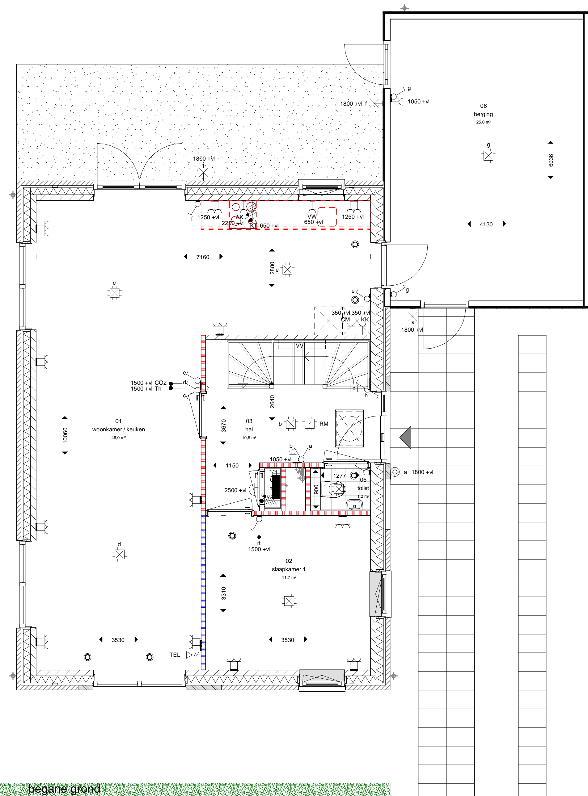
begane grond 1:50
