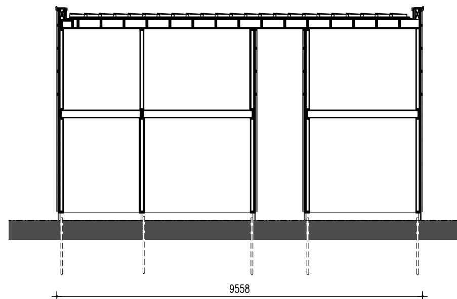
PRINCIPE DOORSNEDE
