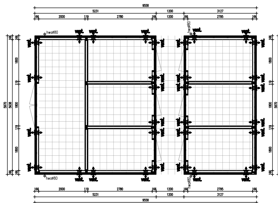
Begane grond
