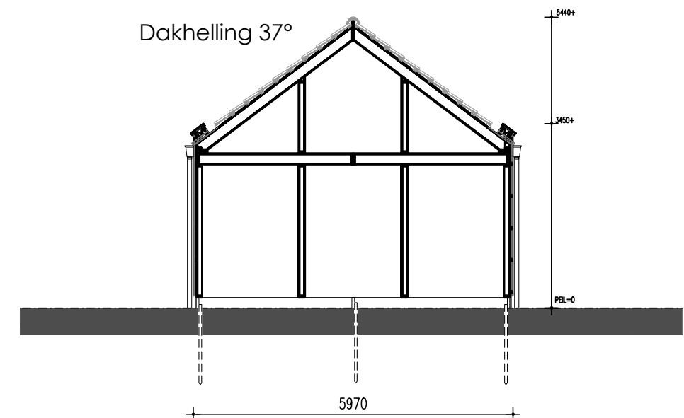
PRINCIPE DOORSNEDE
