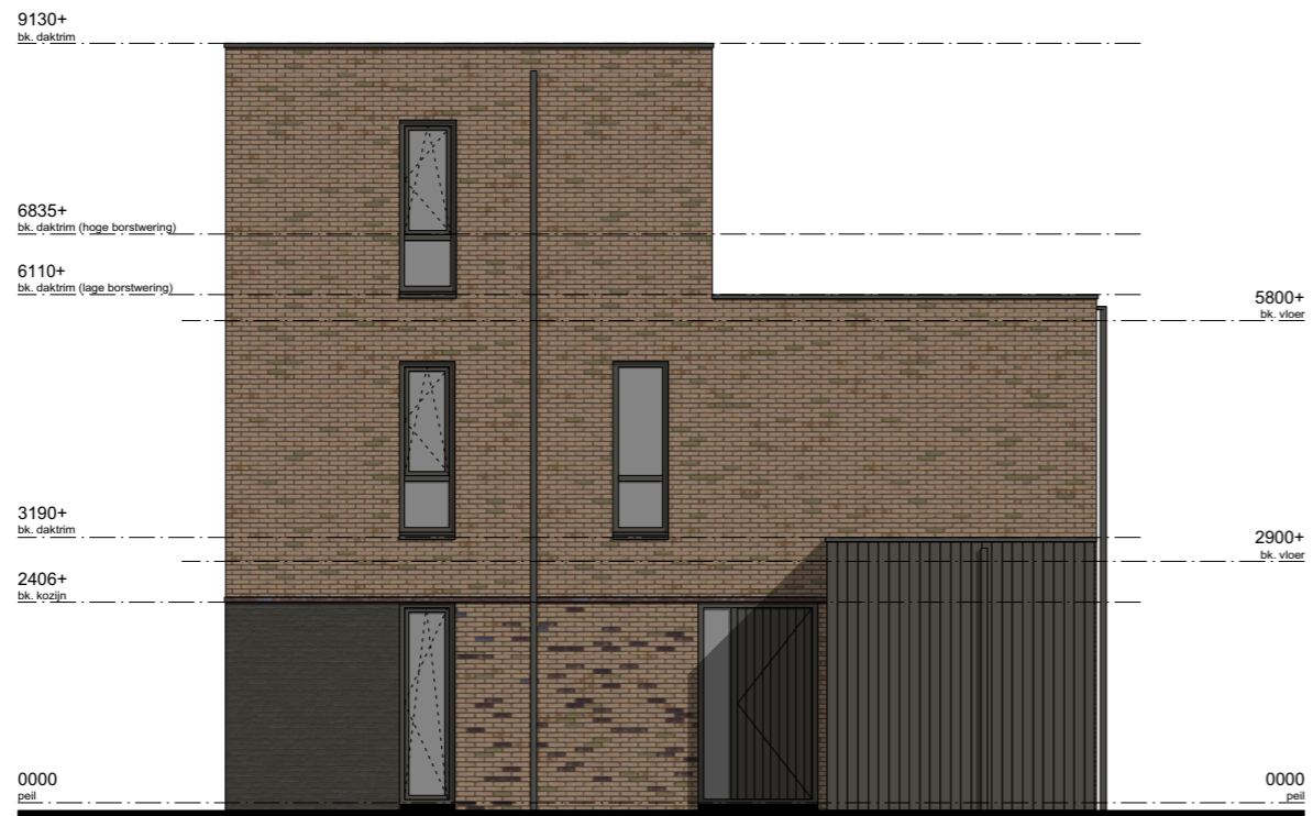
ZIJGEVEL
