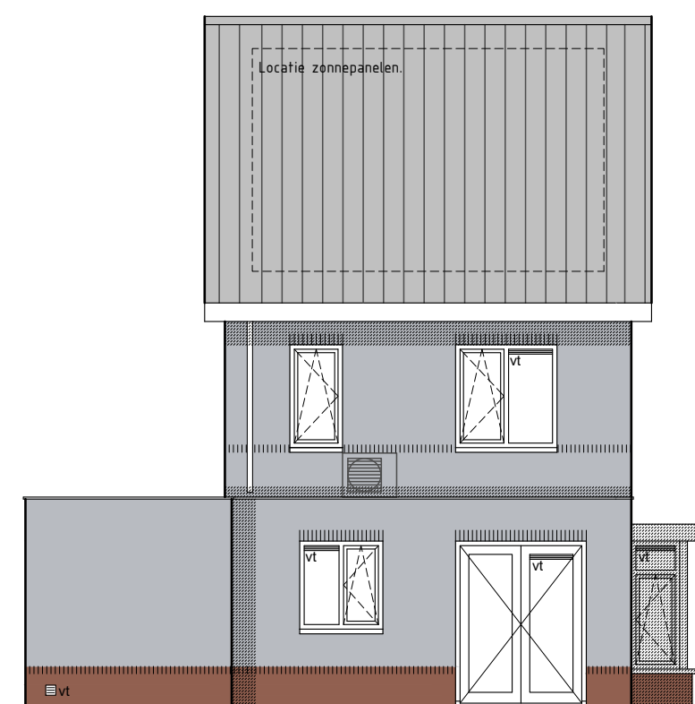
type A3 Achtergevel
