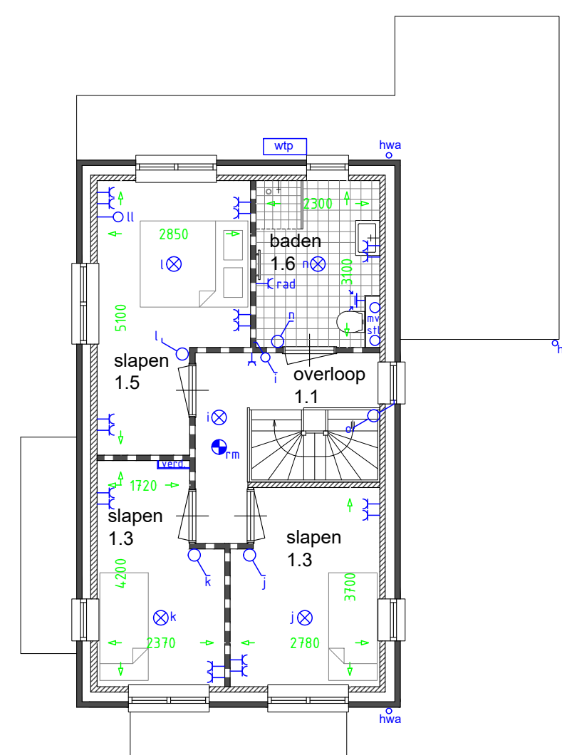
type A3 Verdieping
