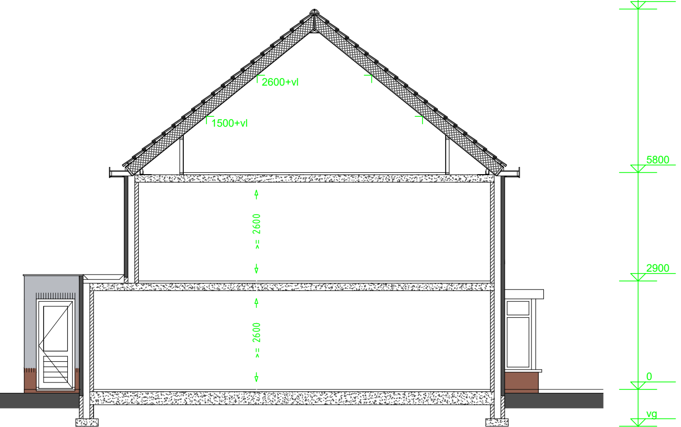
Doorsnede
