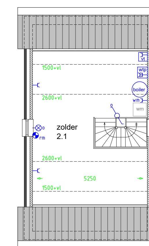
type A3 Zolder
