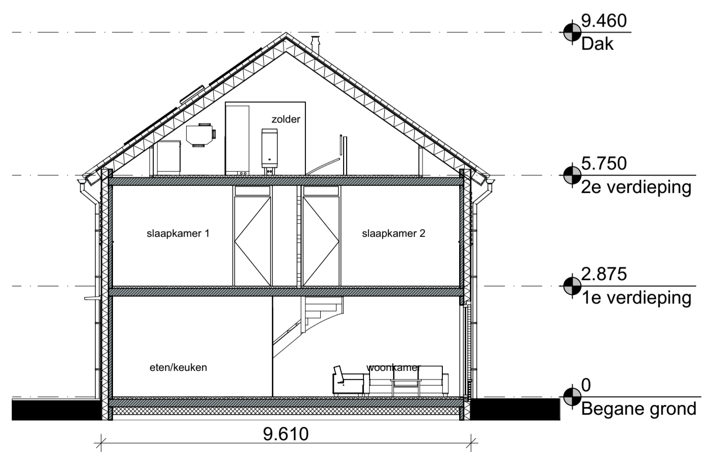
Doorsnede
