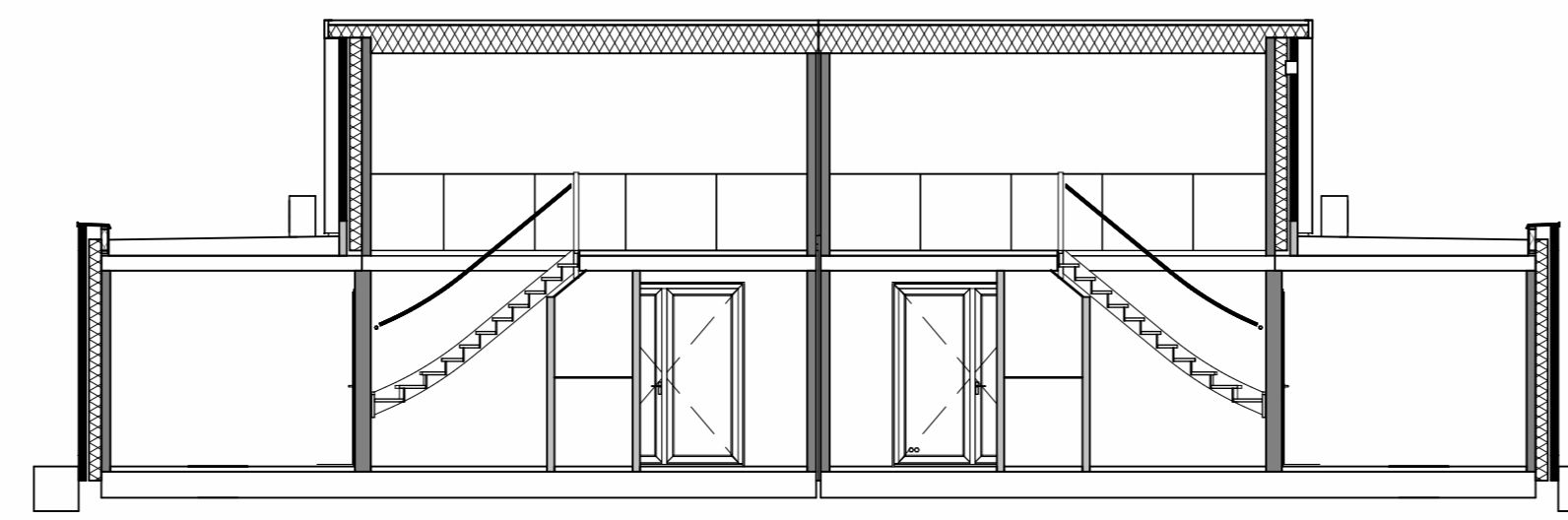
Doorsnede 1 Bnr 17/18 Schaal: 1 : 100
