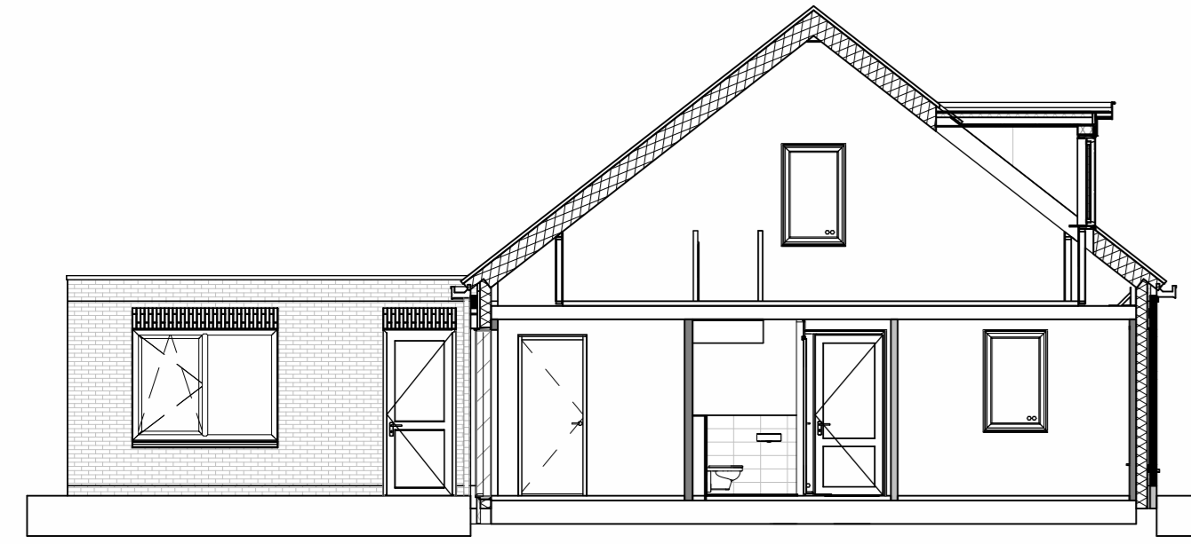
Doorsnede 2 Bnr 17/18 Schaal: 1 : 100
