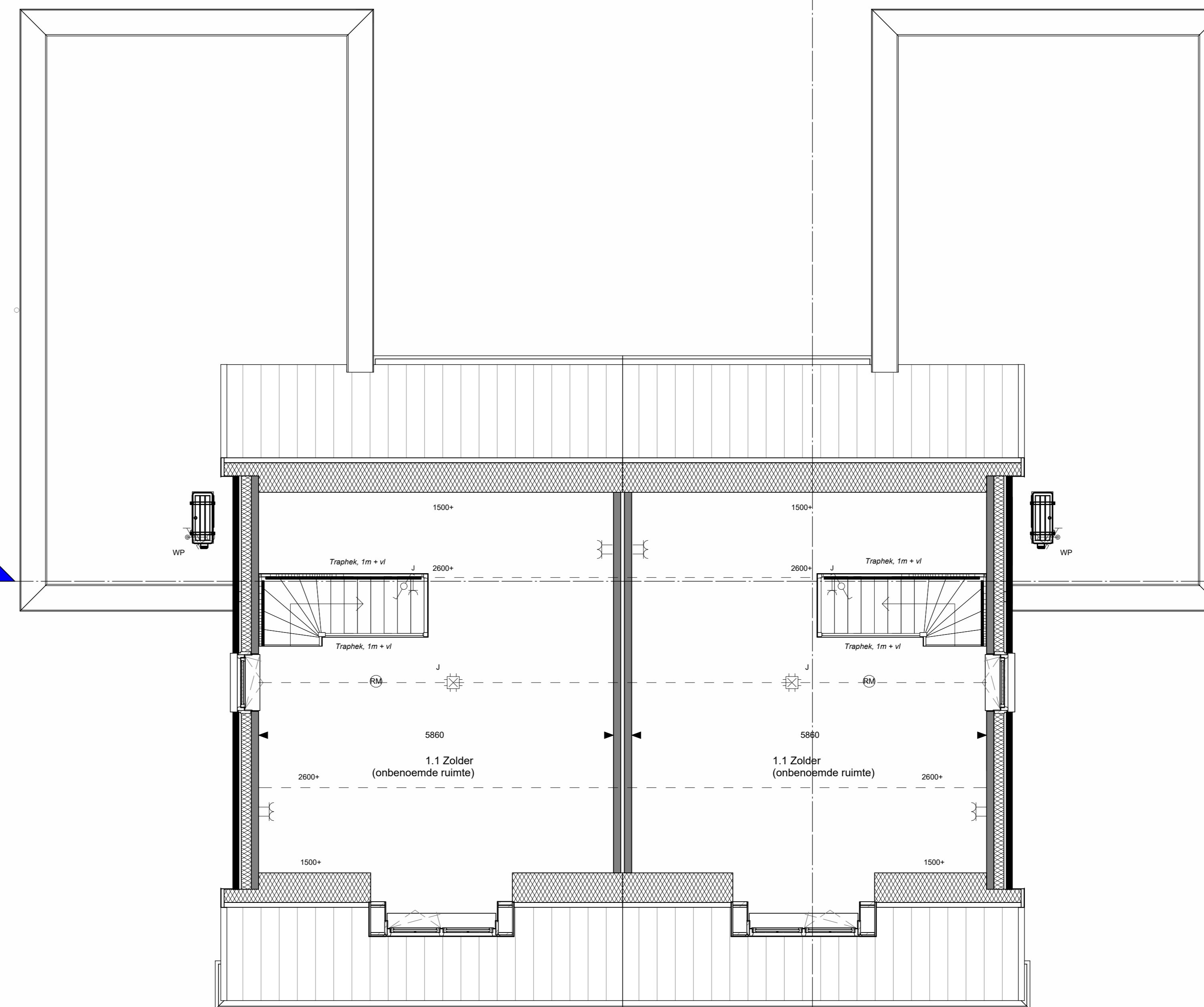
Eerste verdieping Bnr 17/18 Schaal: 1 : 50
