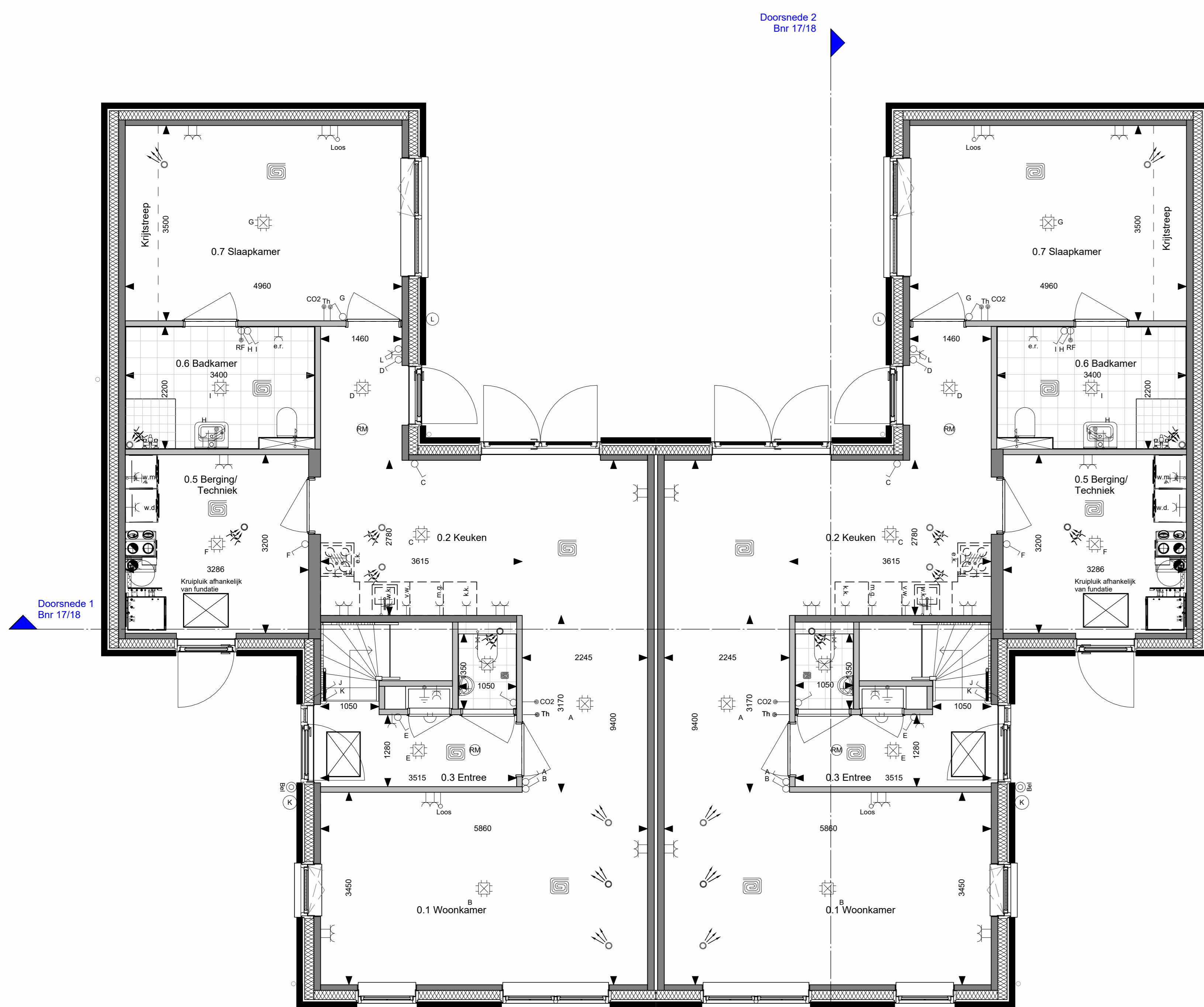
Begane grond Bnr 17/18 Schaal: 1 : 50
