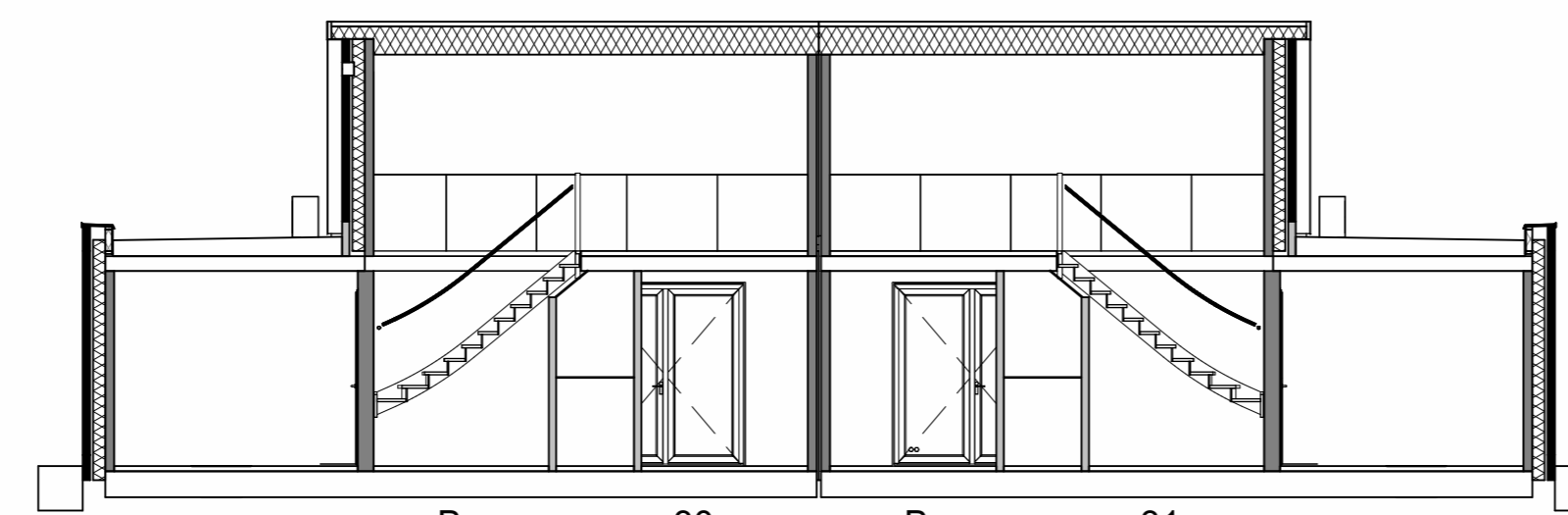
Doorsnede 1 Bnr 30/31 Schaal: 1 : 100
