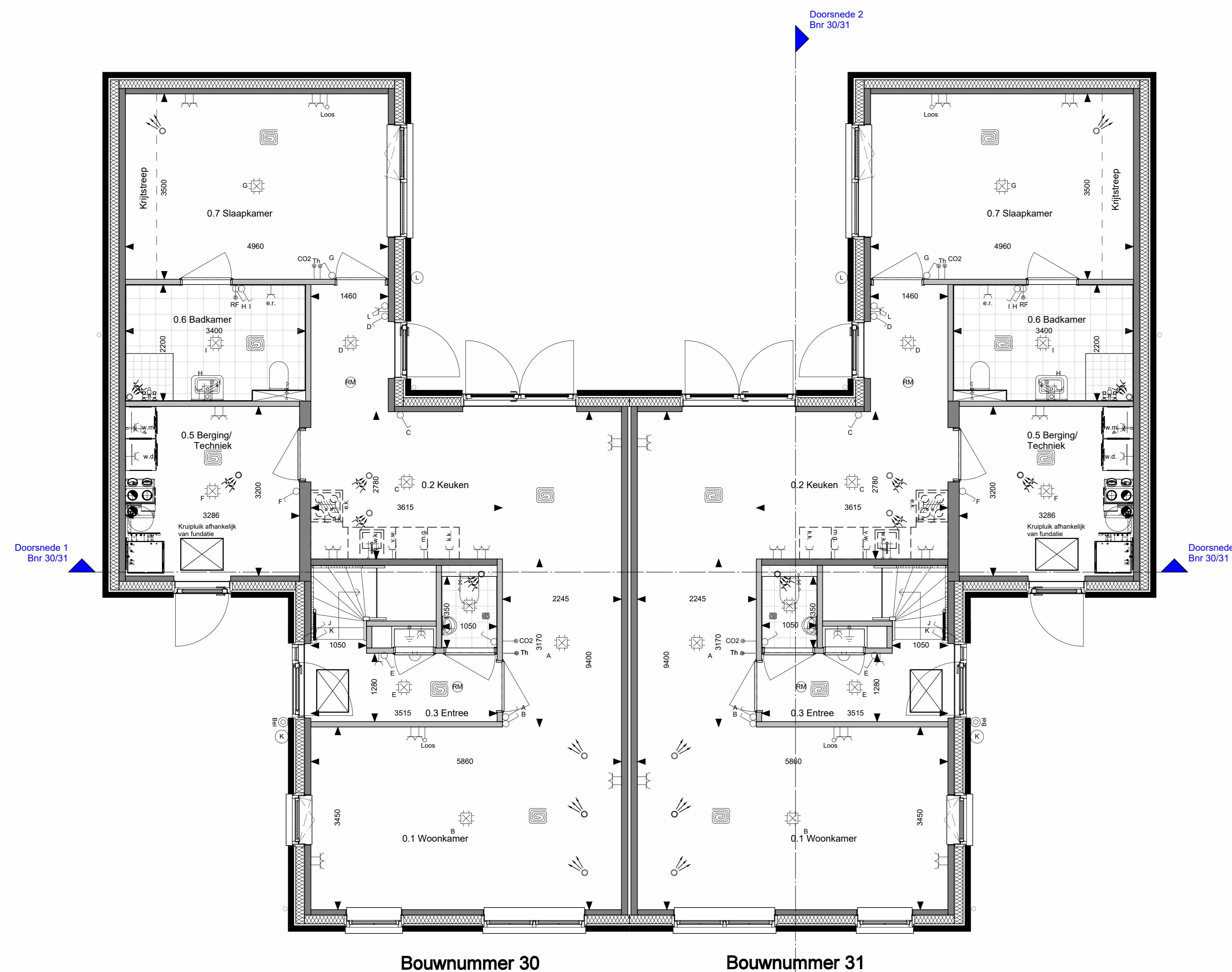
Begane grond Bnr 30/31 Schaal: 1 : 50
