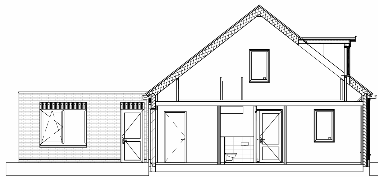
Doorsnede 2 Bnr 30/31 Schaal: 1 : 100
