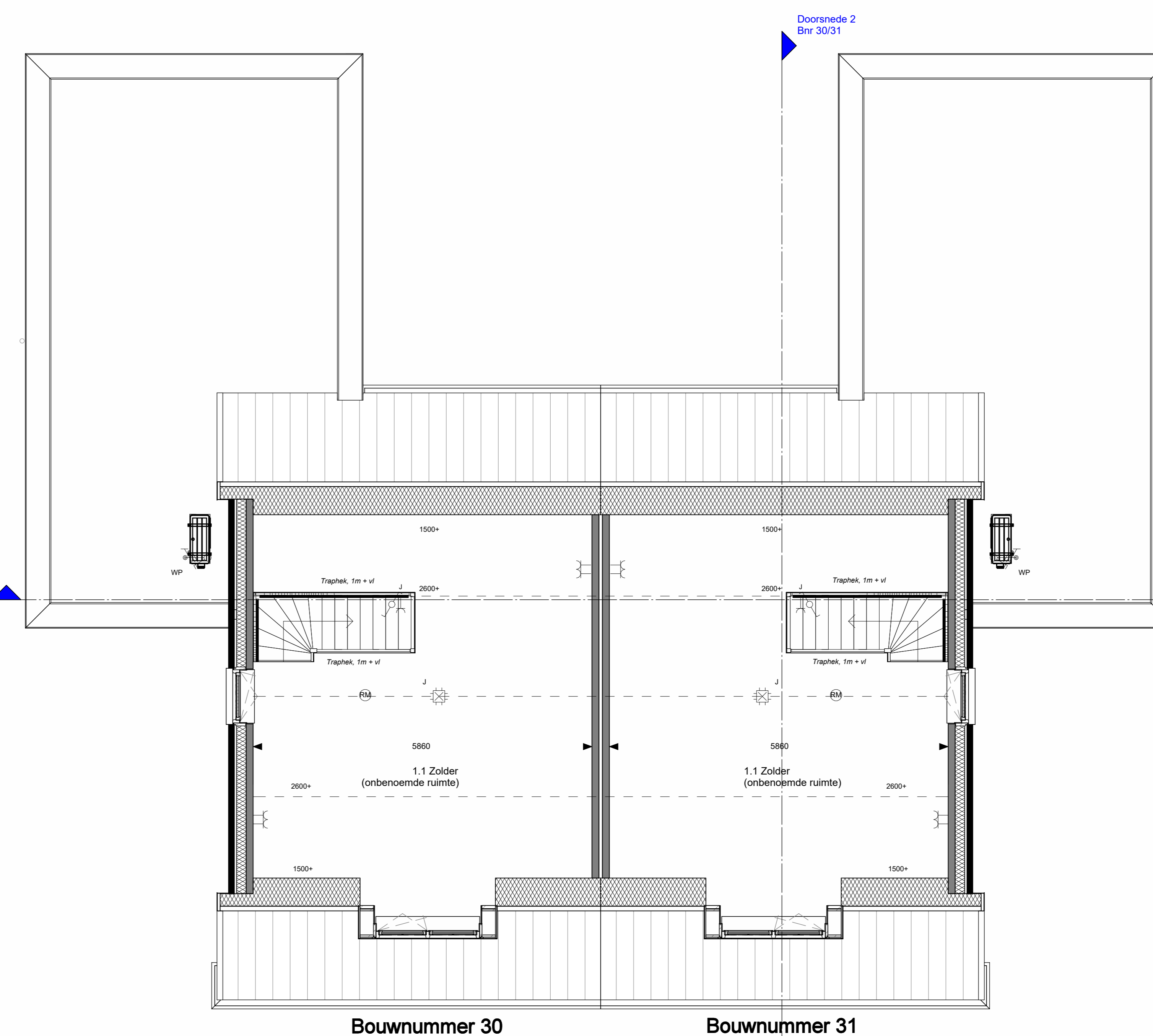
Eerste verdieping Bnr 30/31 Schaal: 1 : 50
