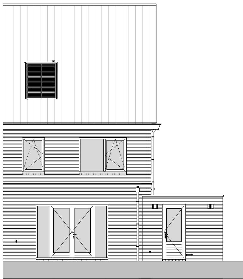
achtergevel 1:100
