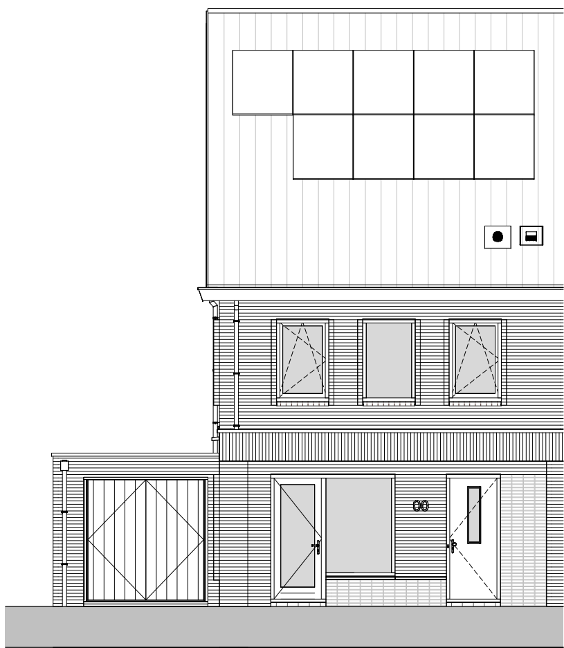
voorgevel 1:100
