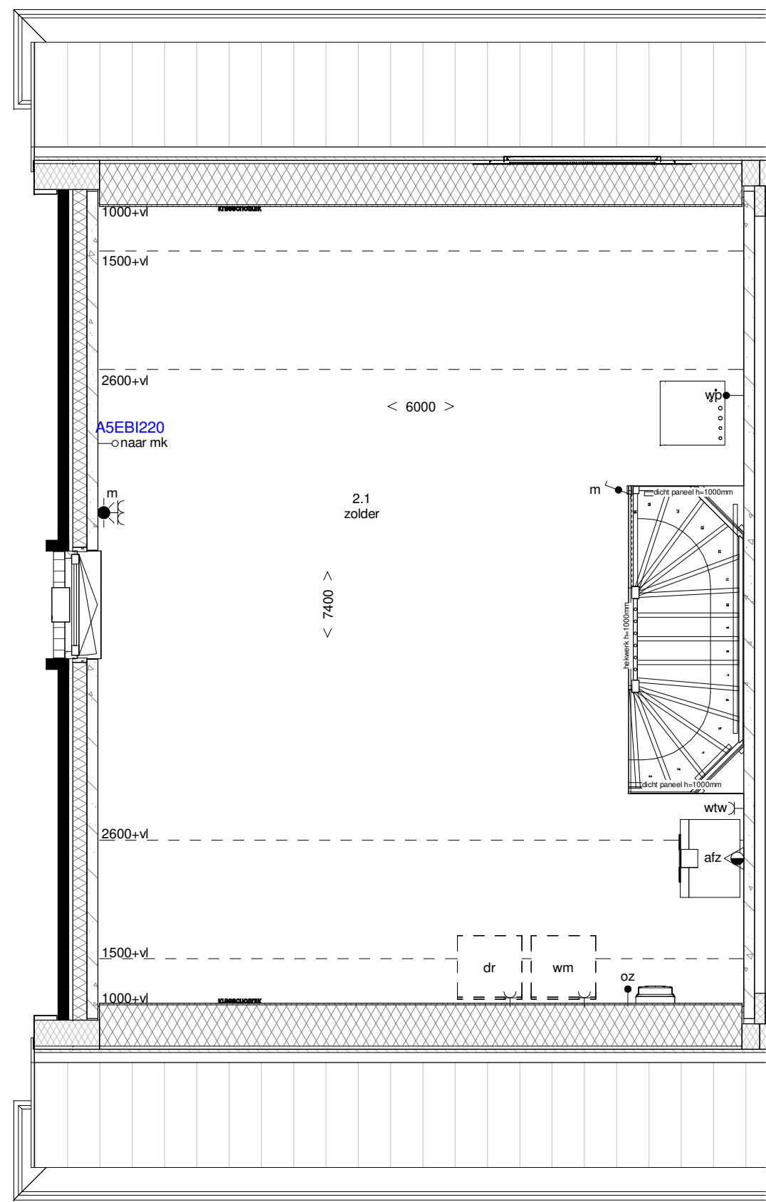
tweede verdieping 1:50
