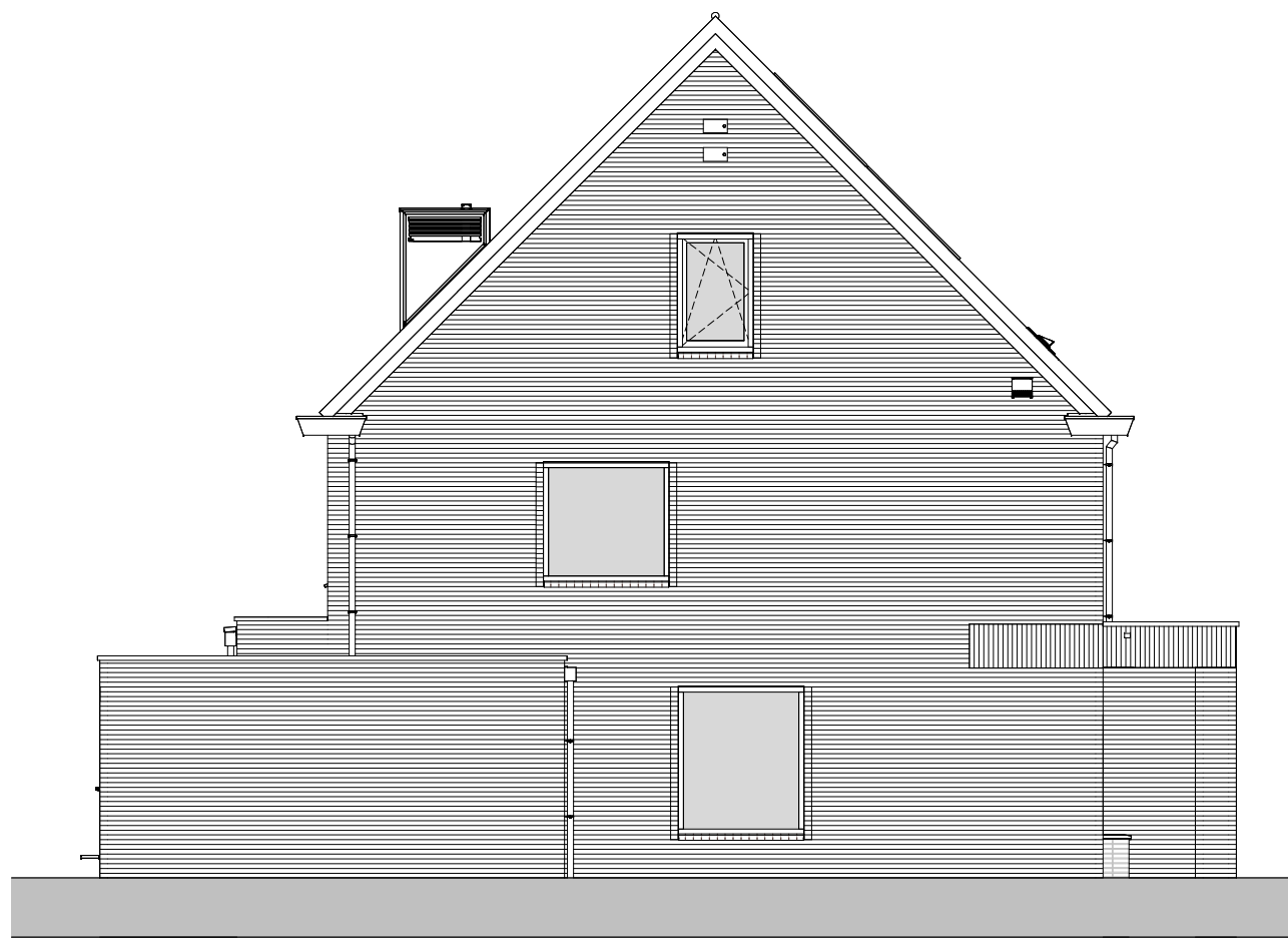
linkergevel 1:100
