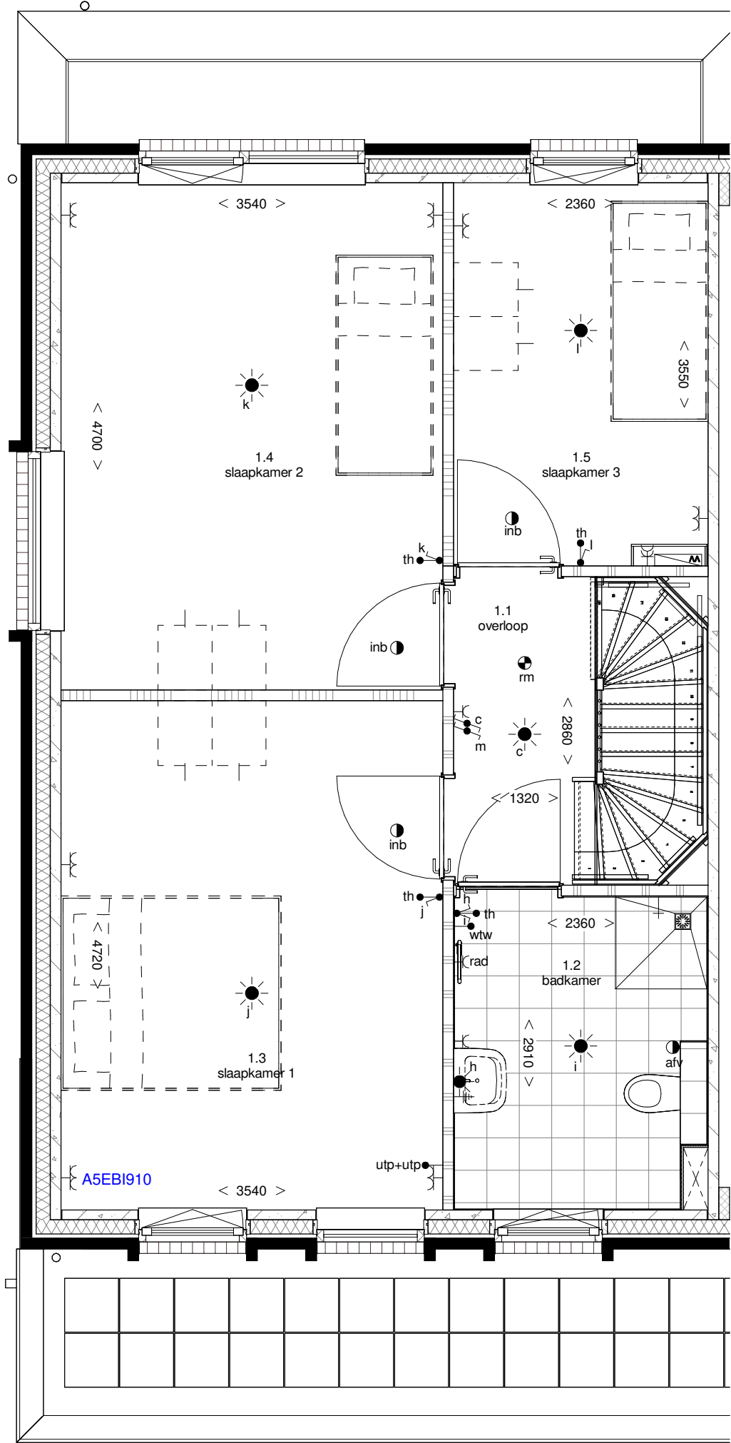
eerste verdieping 1:50
