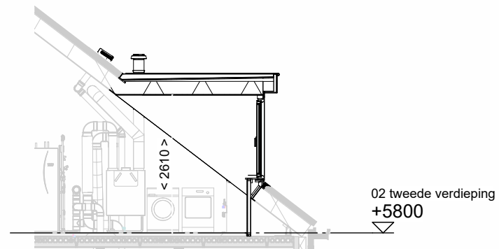
Doorsnede schaal 1:100
