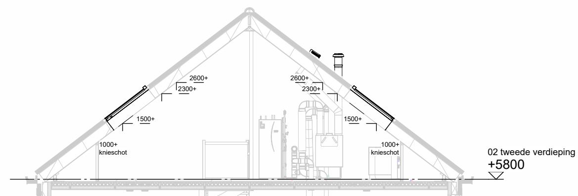
Doorsnede schaal 1:100
