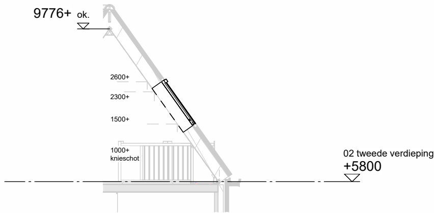
Doorsnede schaal 1:100
