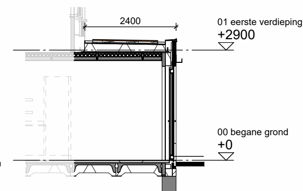
Doorsnede schaal 1:100
