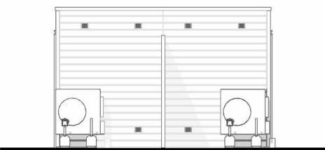
Achtergevel
