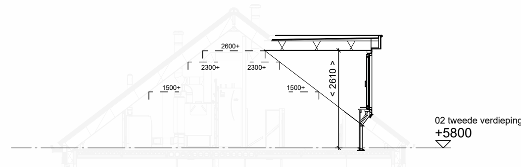
Doorsnede schaal 1:100
