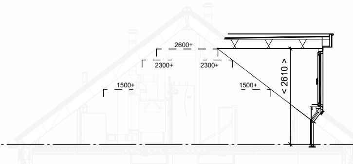
Doorsnede schaal 1:100
