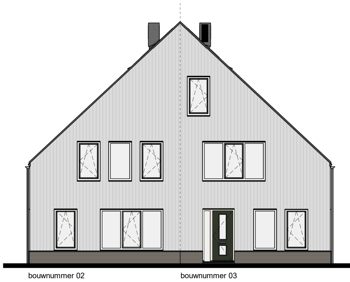
Voorgevel
