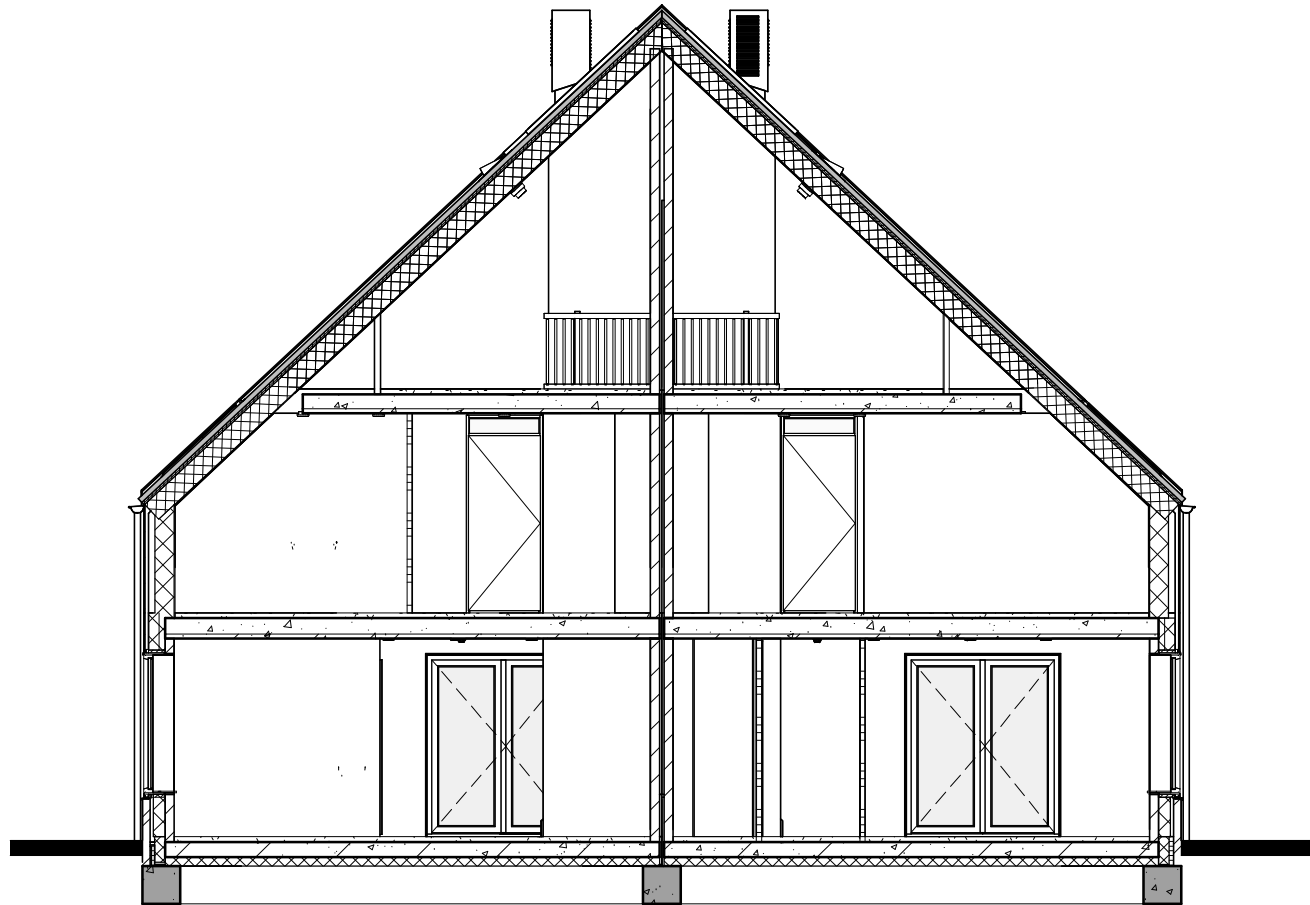
Doorsnede
