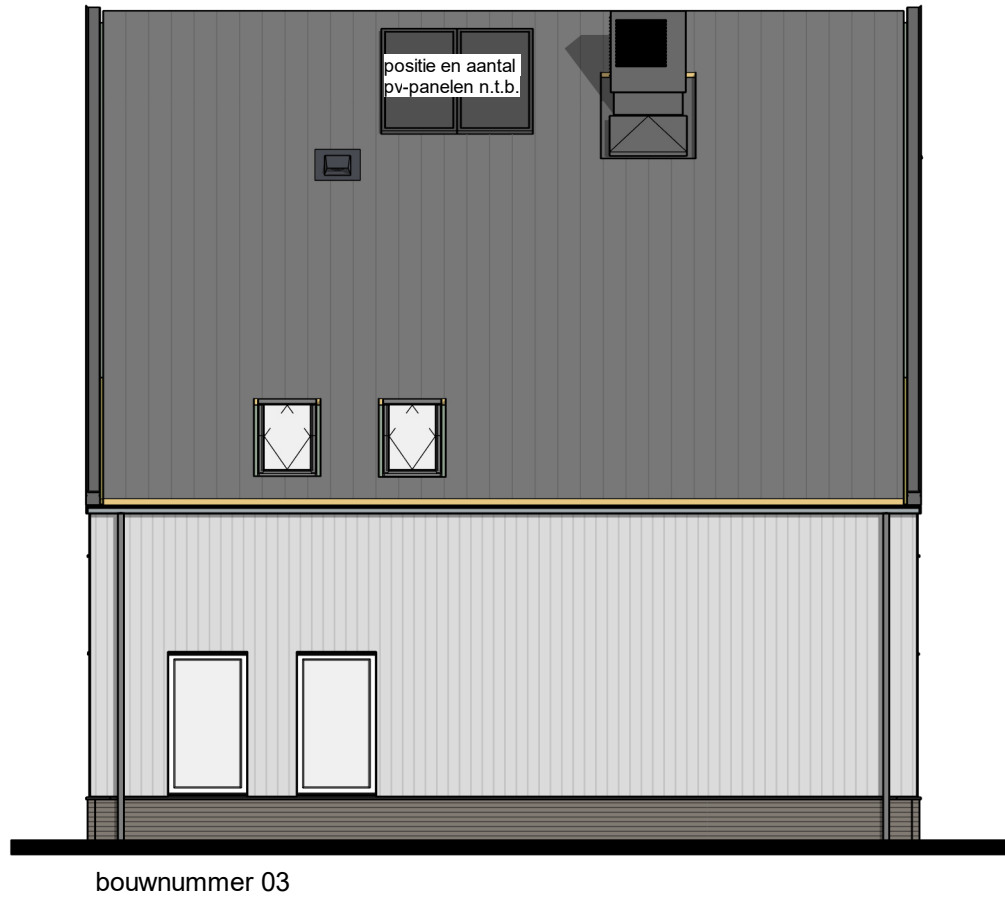
Rechter zijgevel
