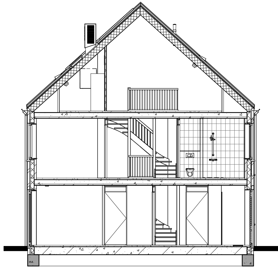
Doorsnede
