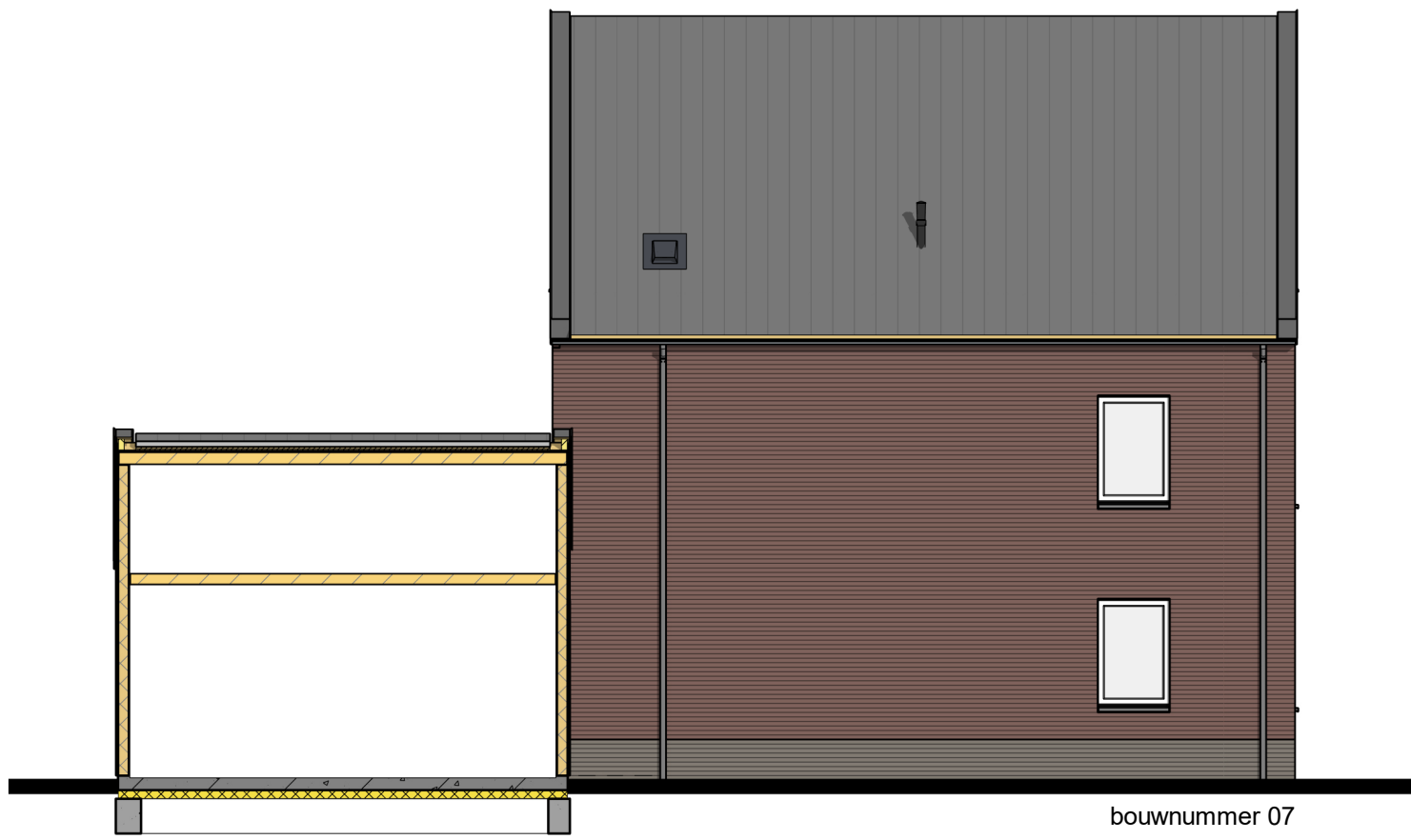
Linker zijgevel
