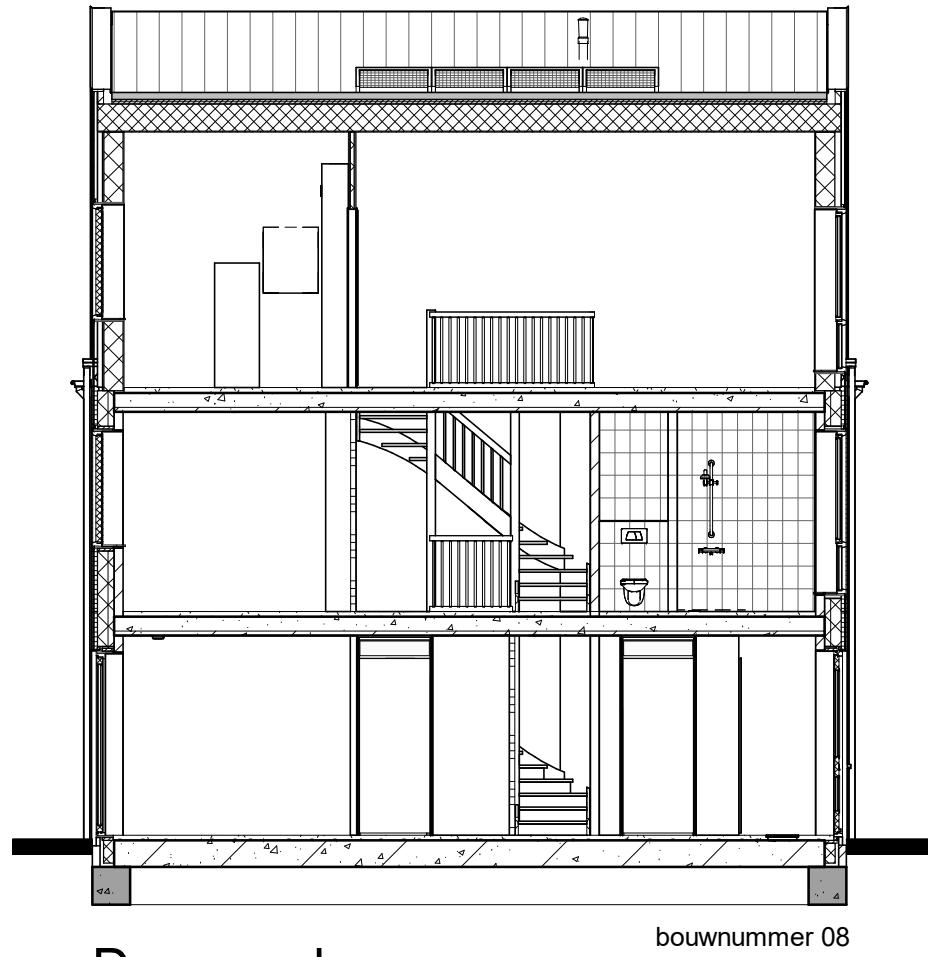
Doorsnede
