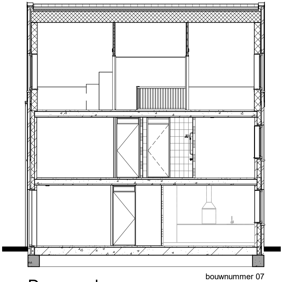
Doorsnede
