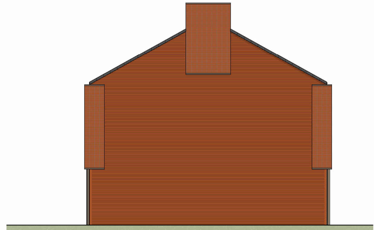
linkergevel
