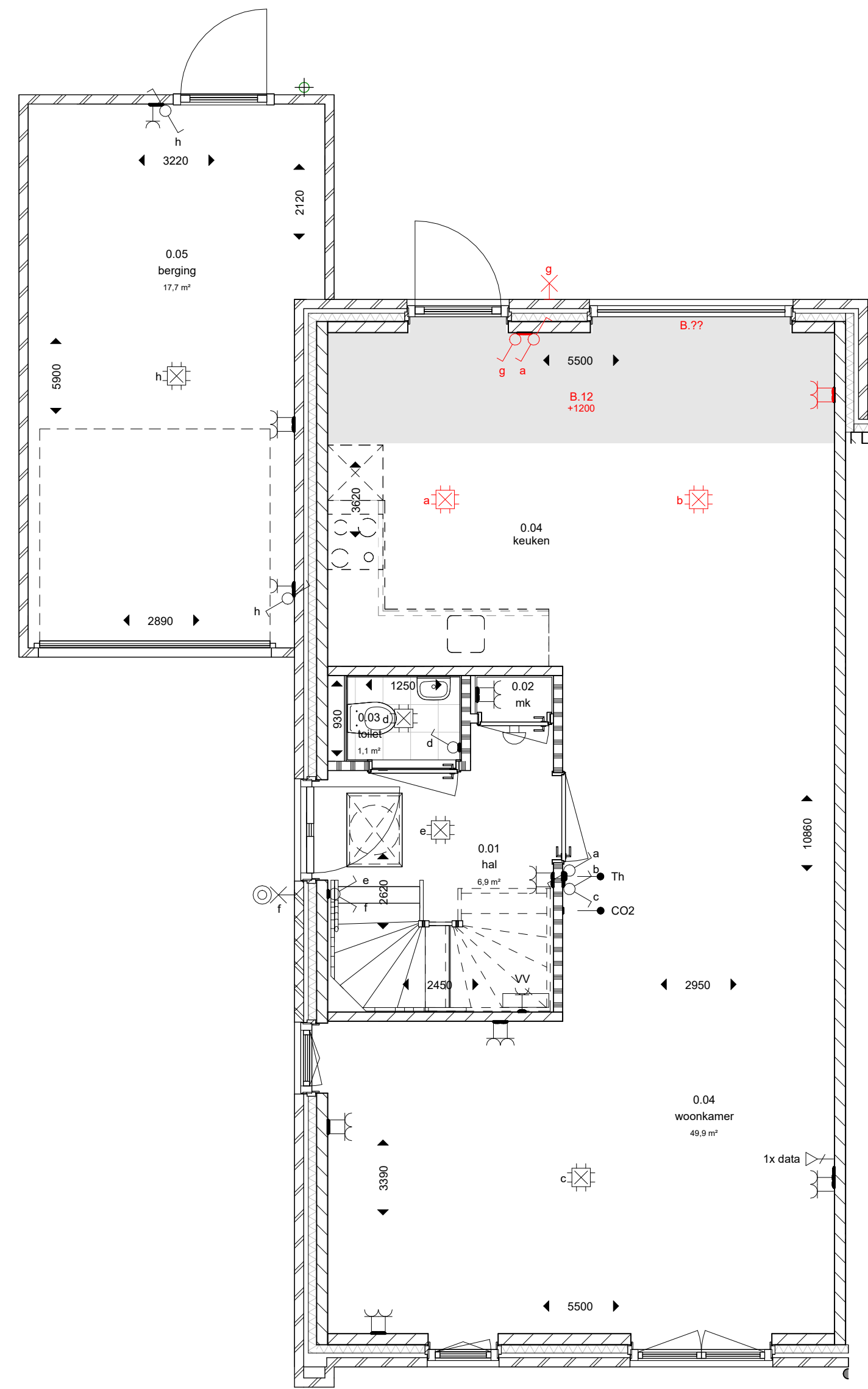
begane grond 1:50
