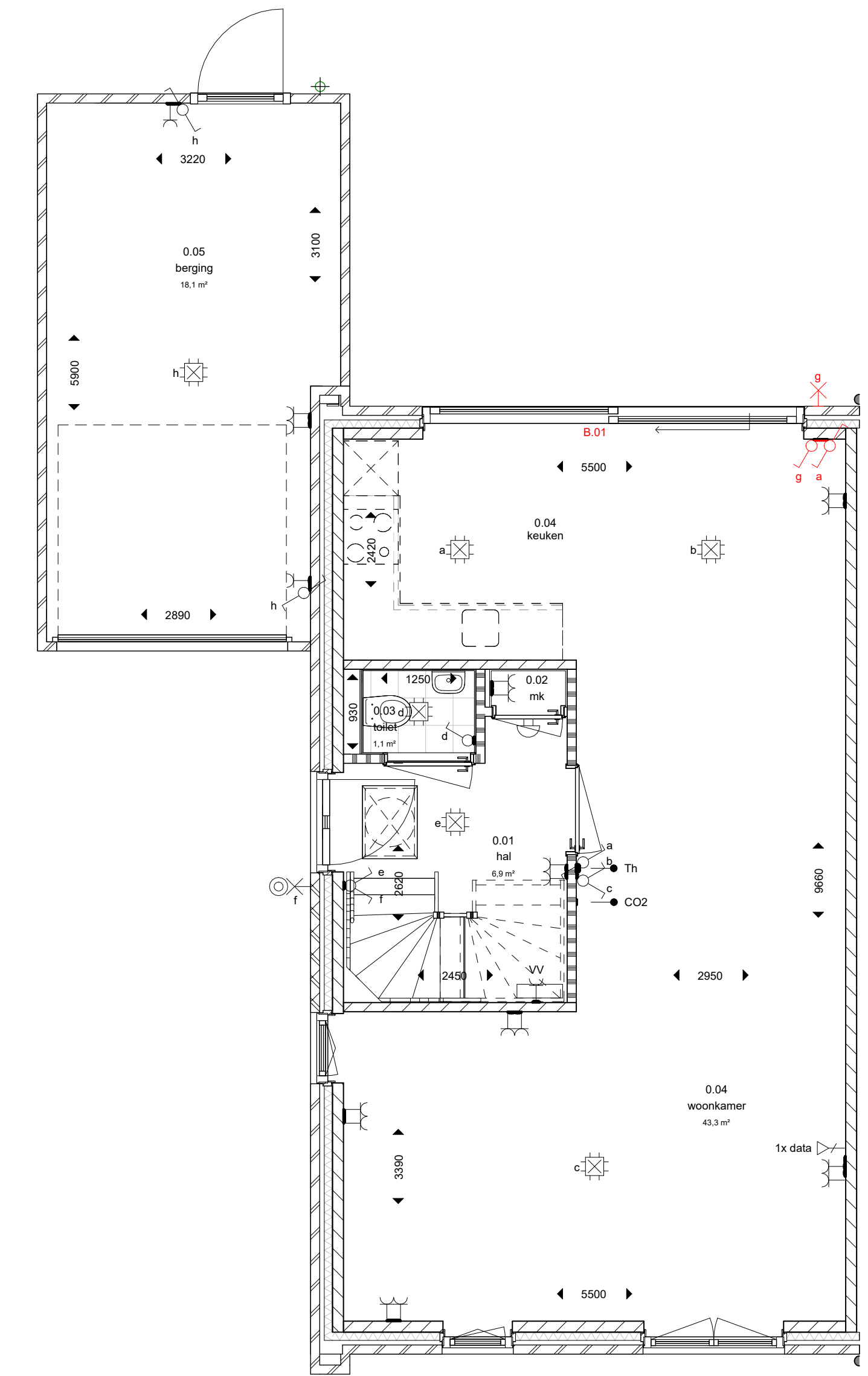
begane grond 1:50
