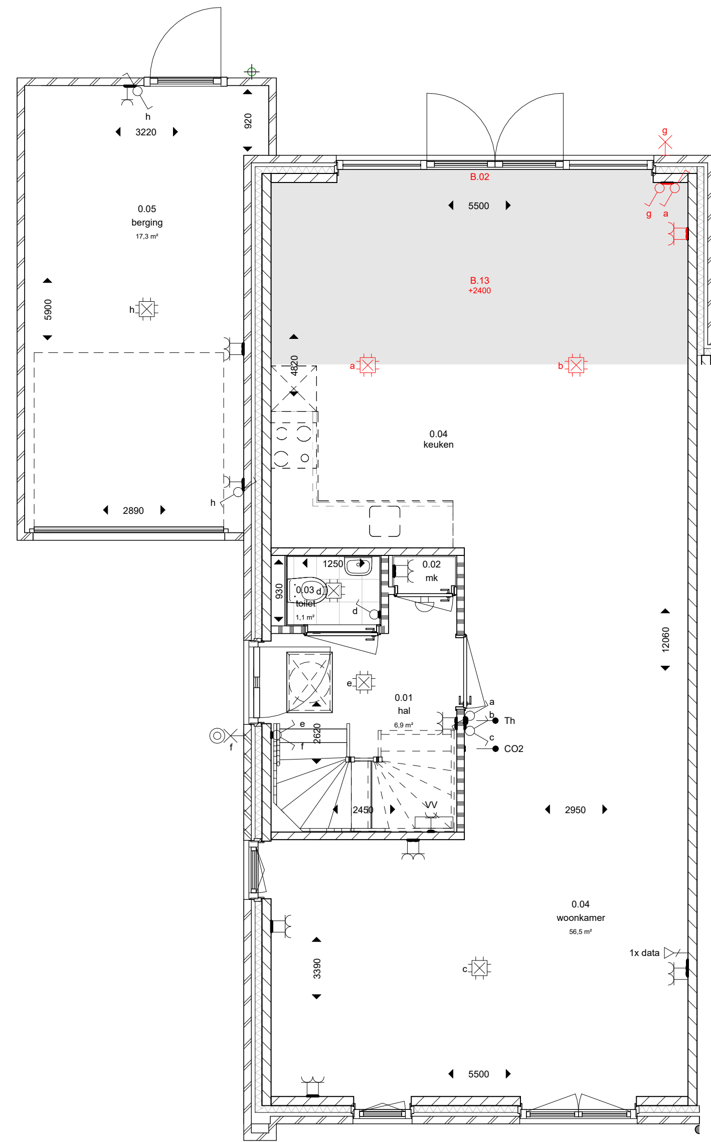
begane grond 1:50
