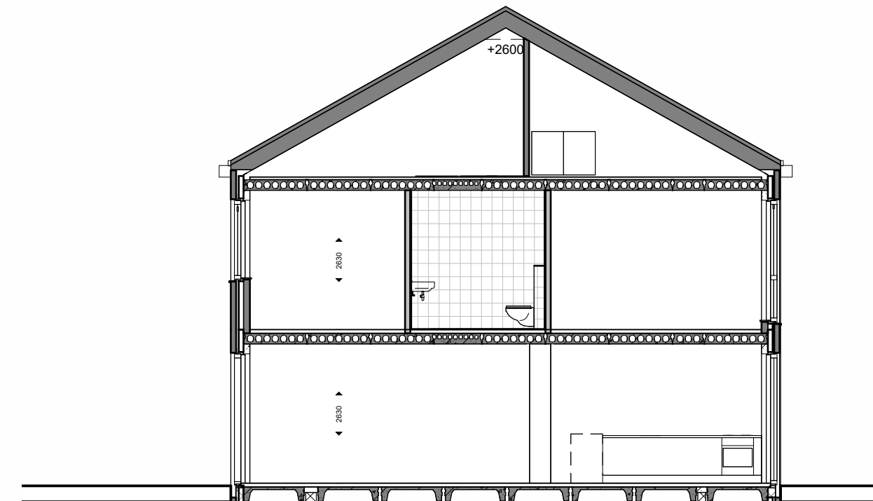
doorsnede 1:100
