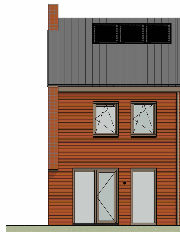
achtergevel 1:100
