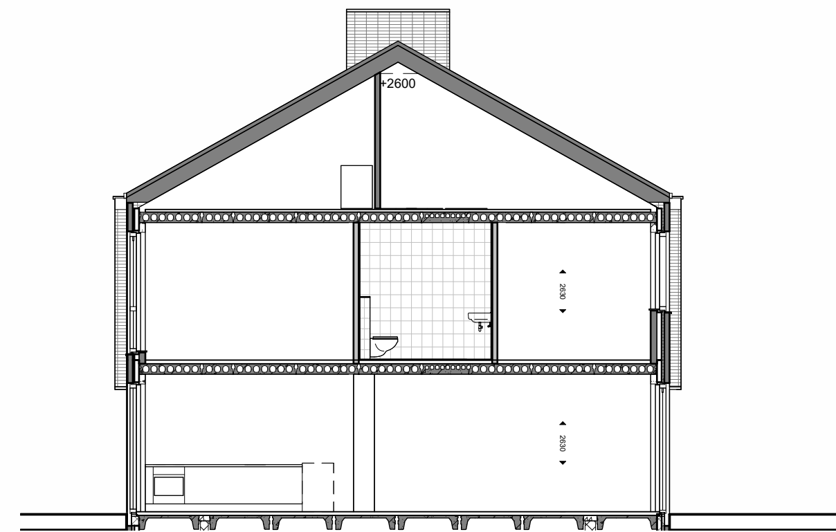
doorsnede 1:100
