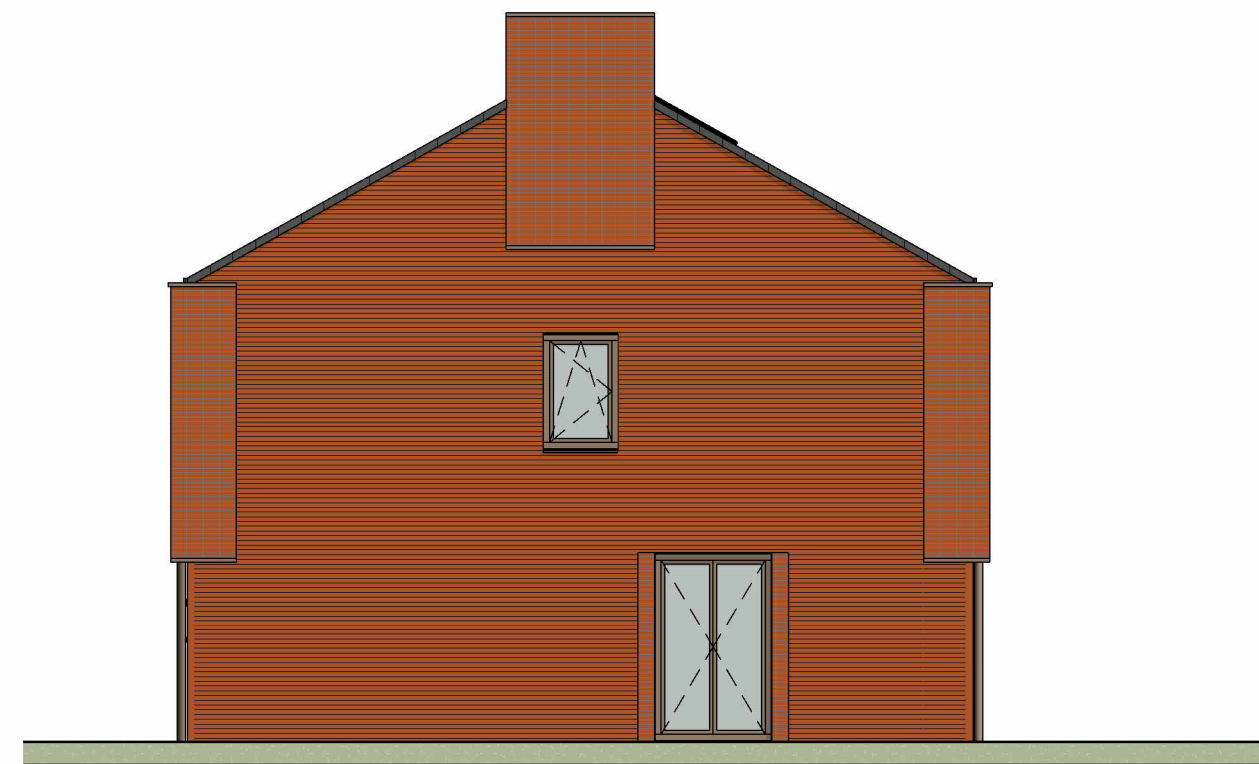
rechtgevel 1:100
