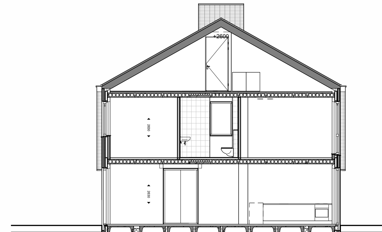
doorsnede 1:100
