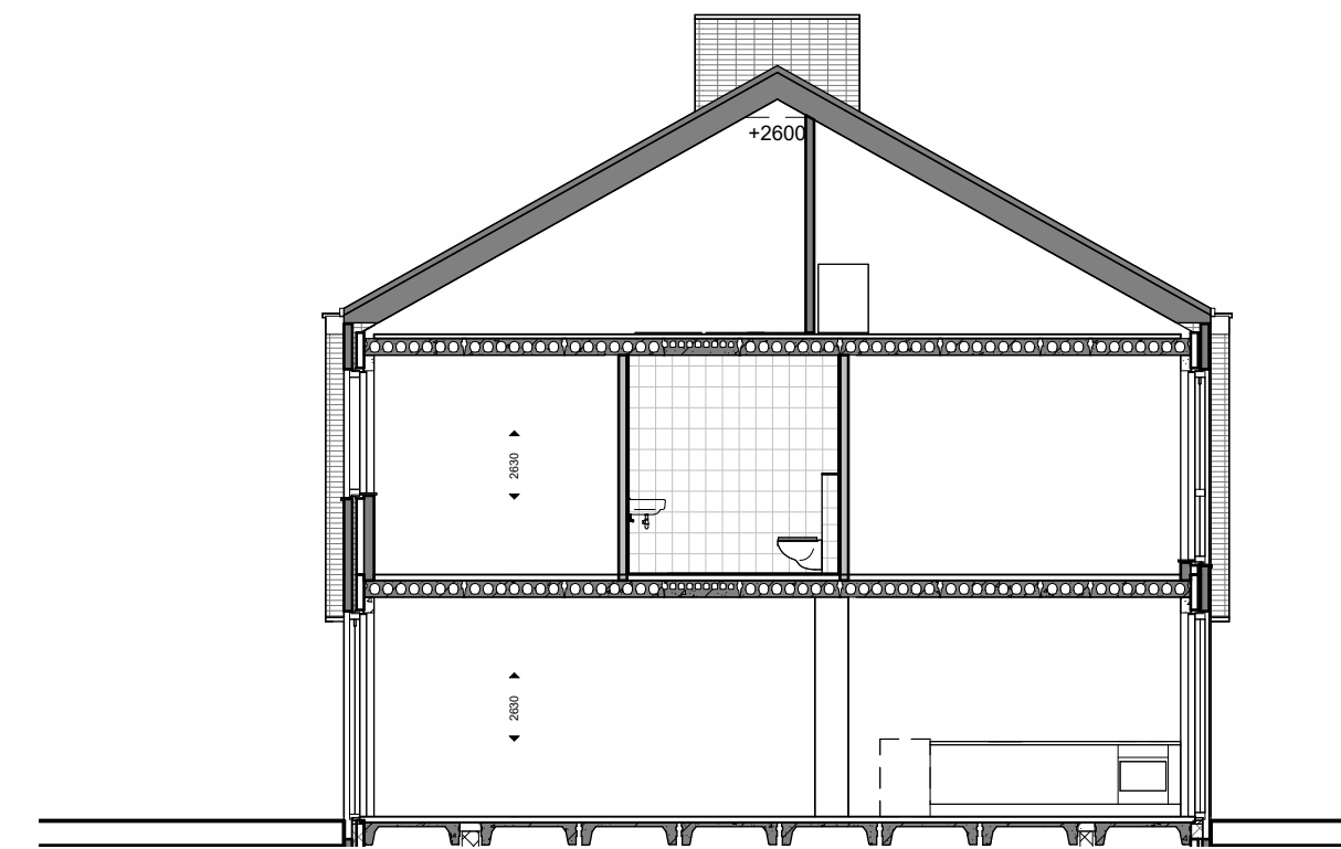
doorsnede 1:100
