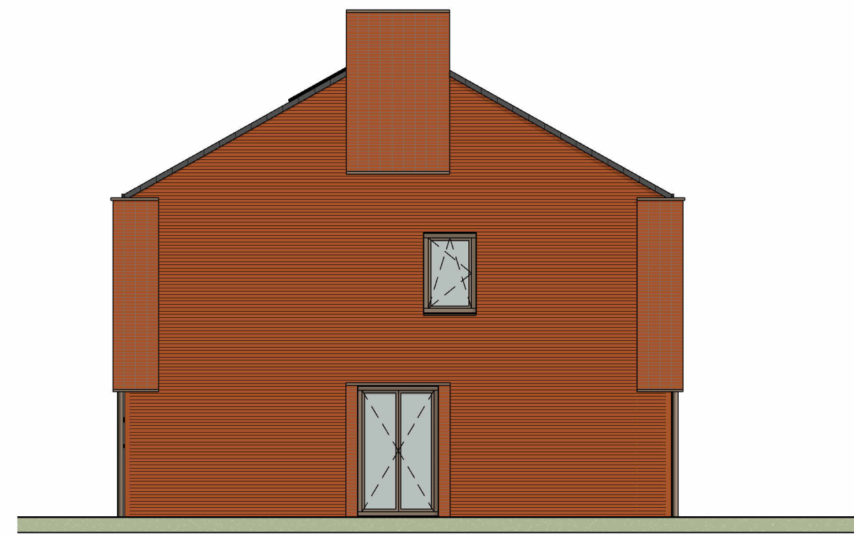
rechtgevel 1: 100
