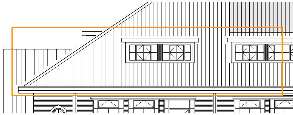
Oostgevel
