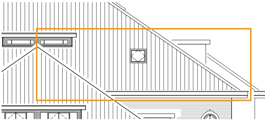
Zuidgevel
