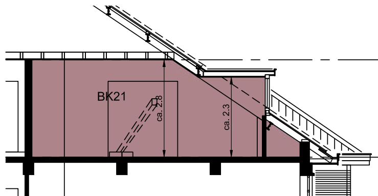
Doorsnede A-A
