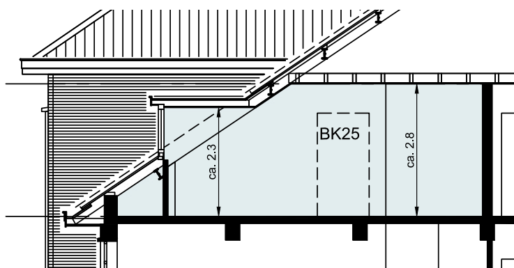
Doorsnede A-A
