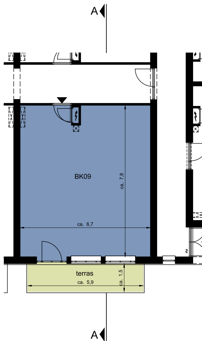
Begane grond
