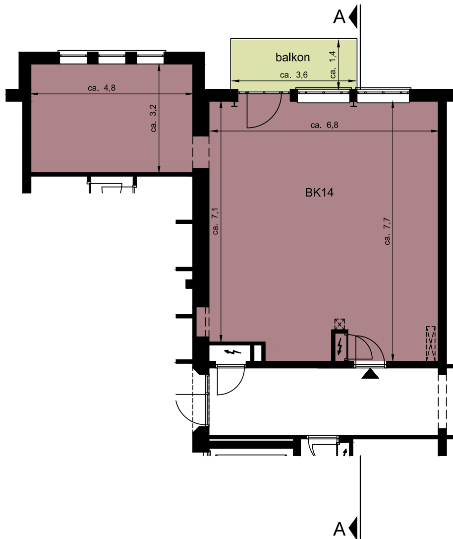
Begane grond
