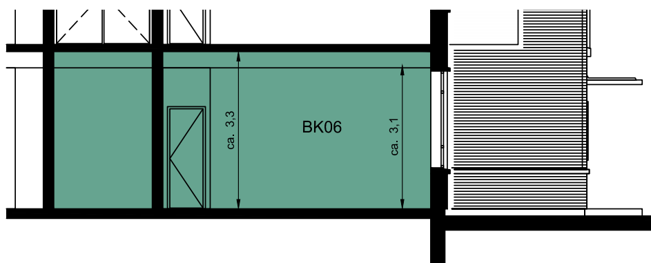
Doorsnede A-A
