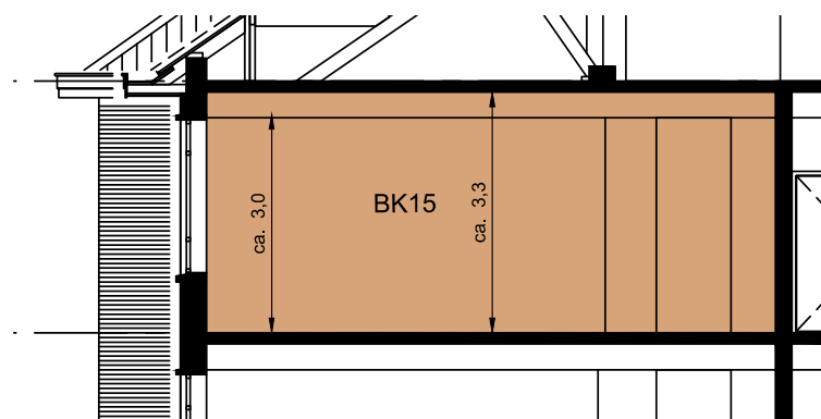
Doorsnede A-A
