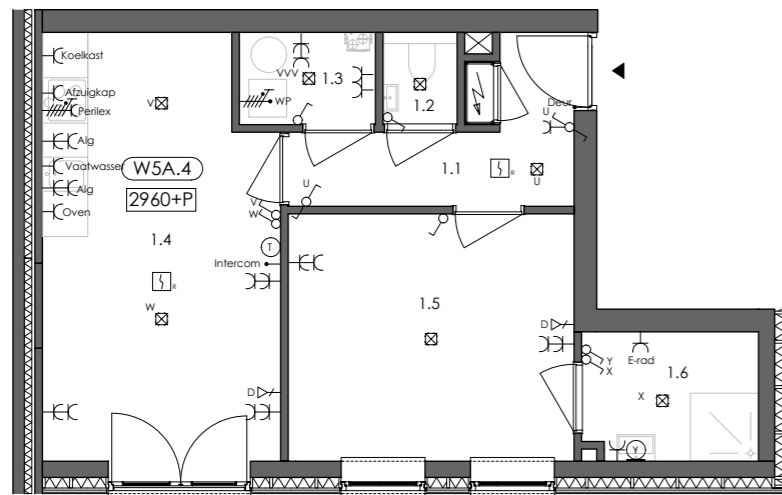
APPARTEMENT W5A.4
