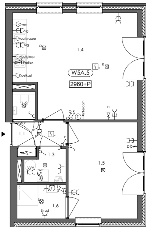
APPARTEMENT W5A.5
