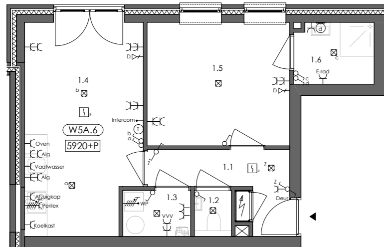
APPARTEMENT W5A.6
