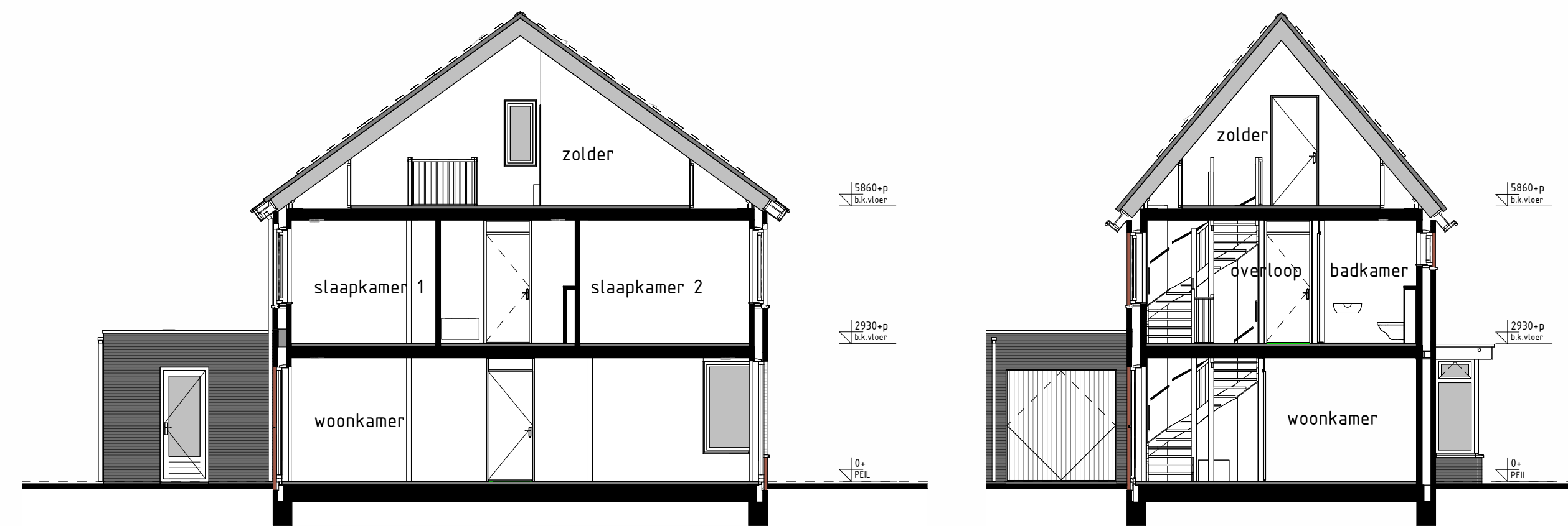
DOORSNEDEN A-A
