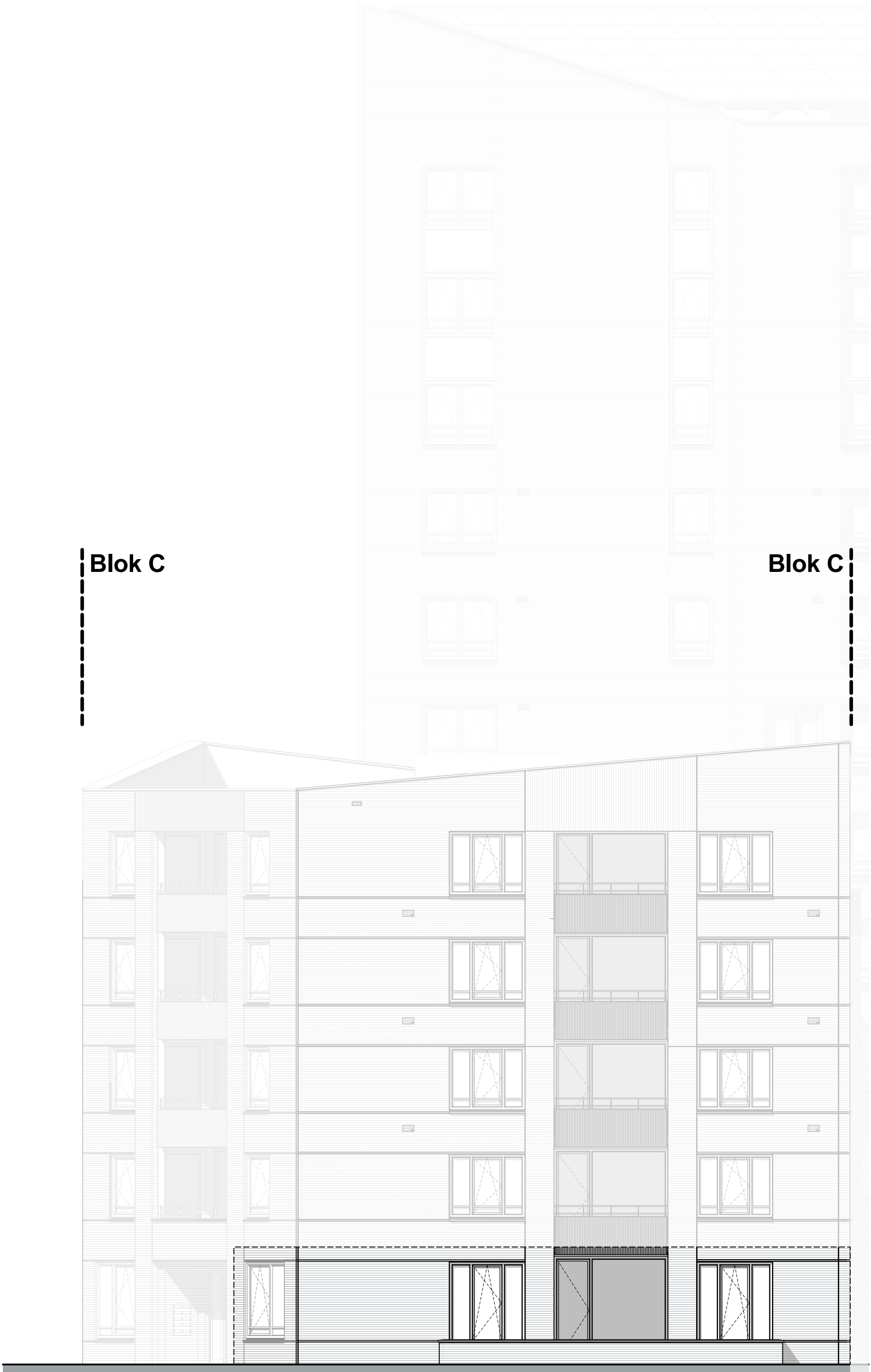
blok C G3 | 1:100
