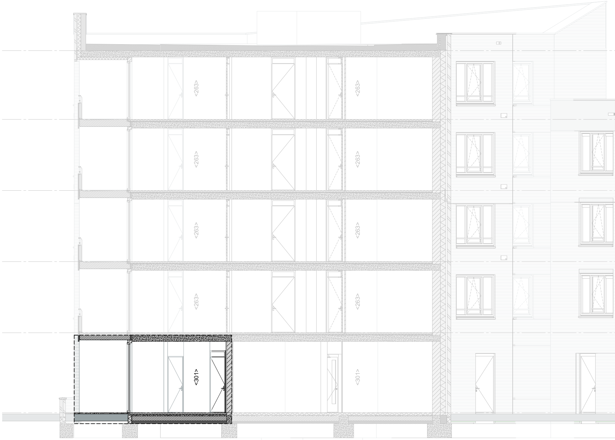
Doorsnede BB | 1:100
