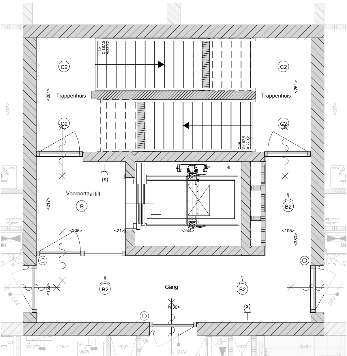
01 eerste verdieping | 1:50
