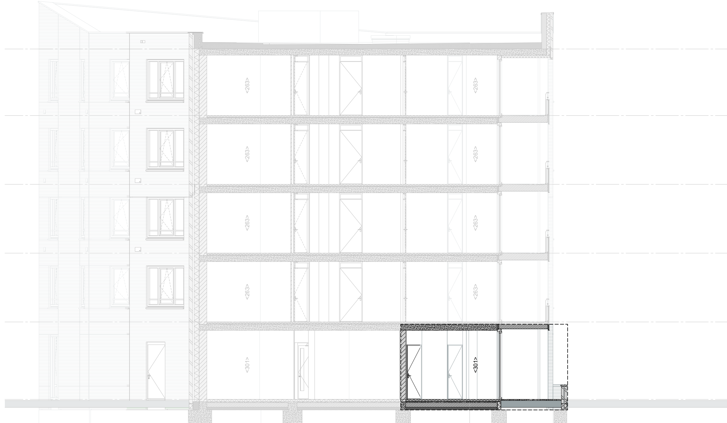
Doorsnede BB | 1:100
