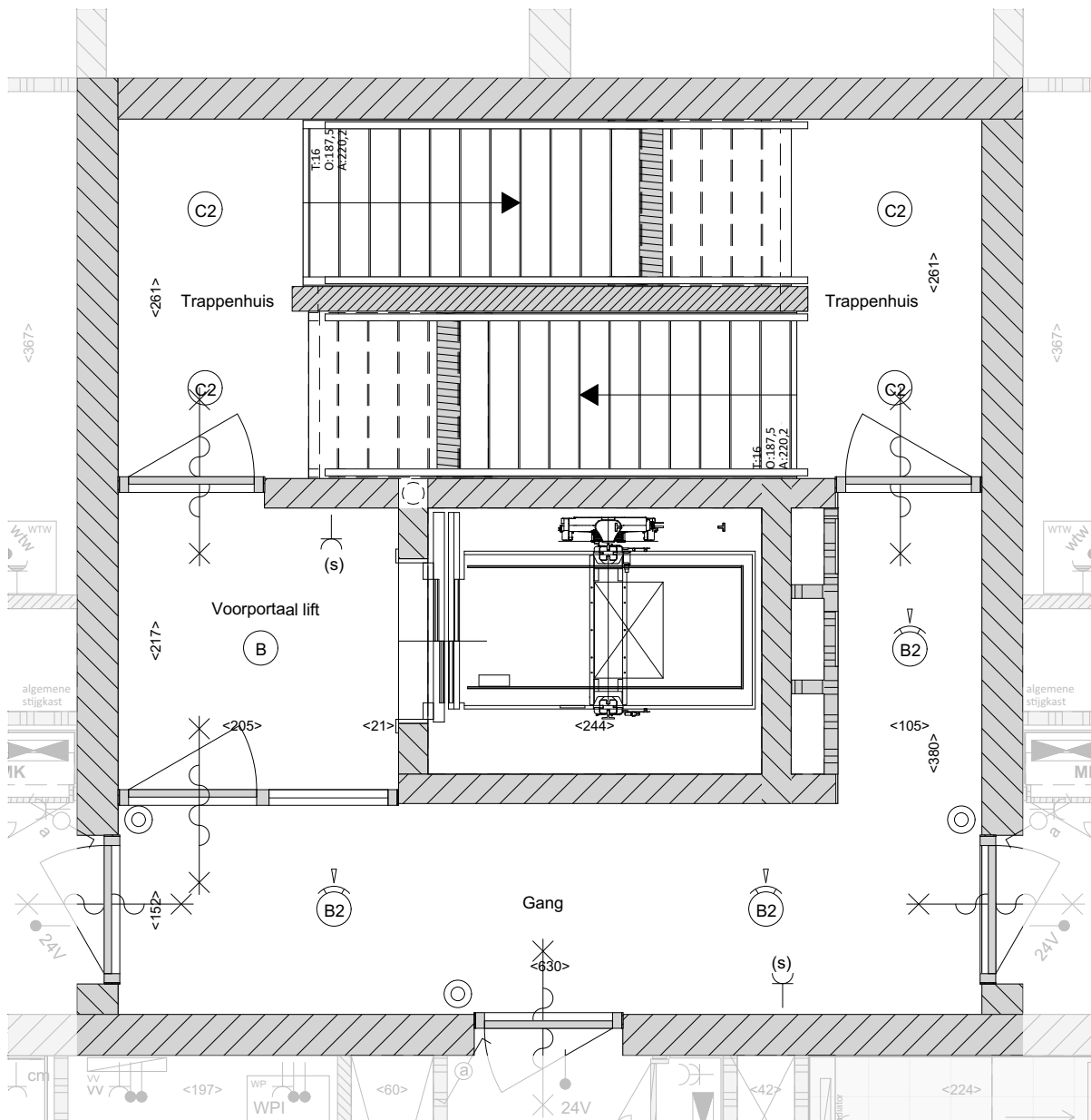
02 tweede verdieping | 1:50
