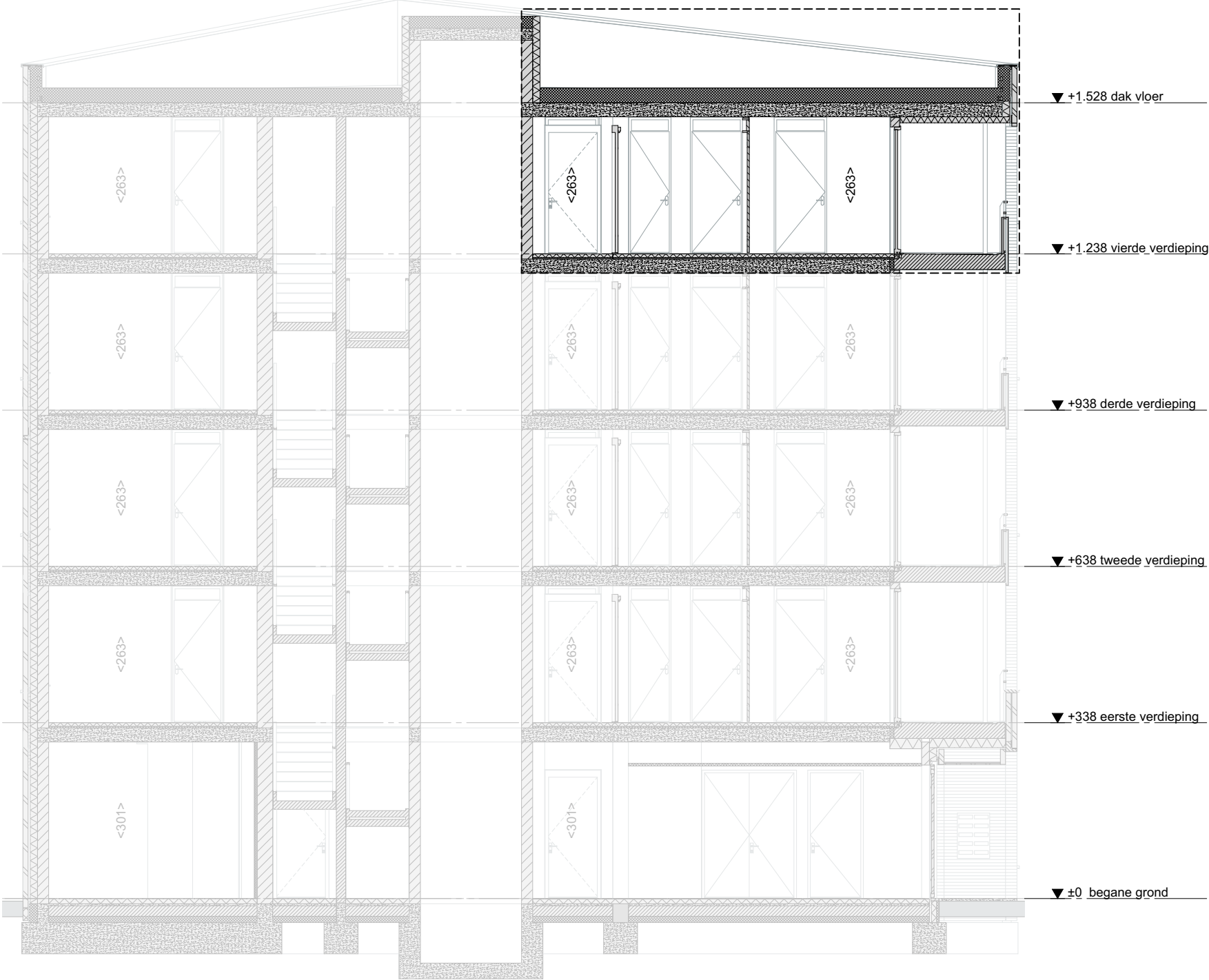
Doorsnede AA | 1:100
