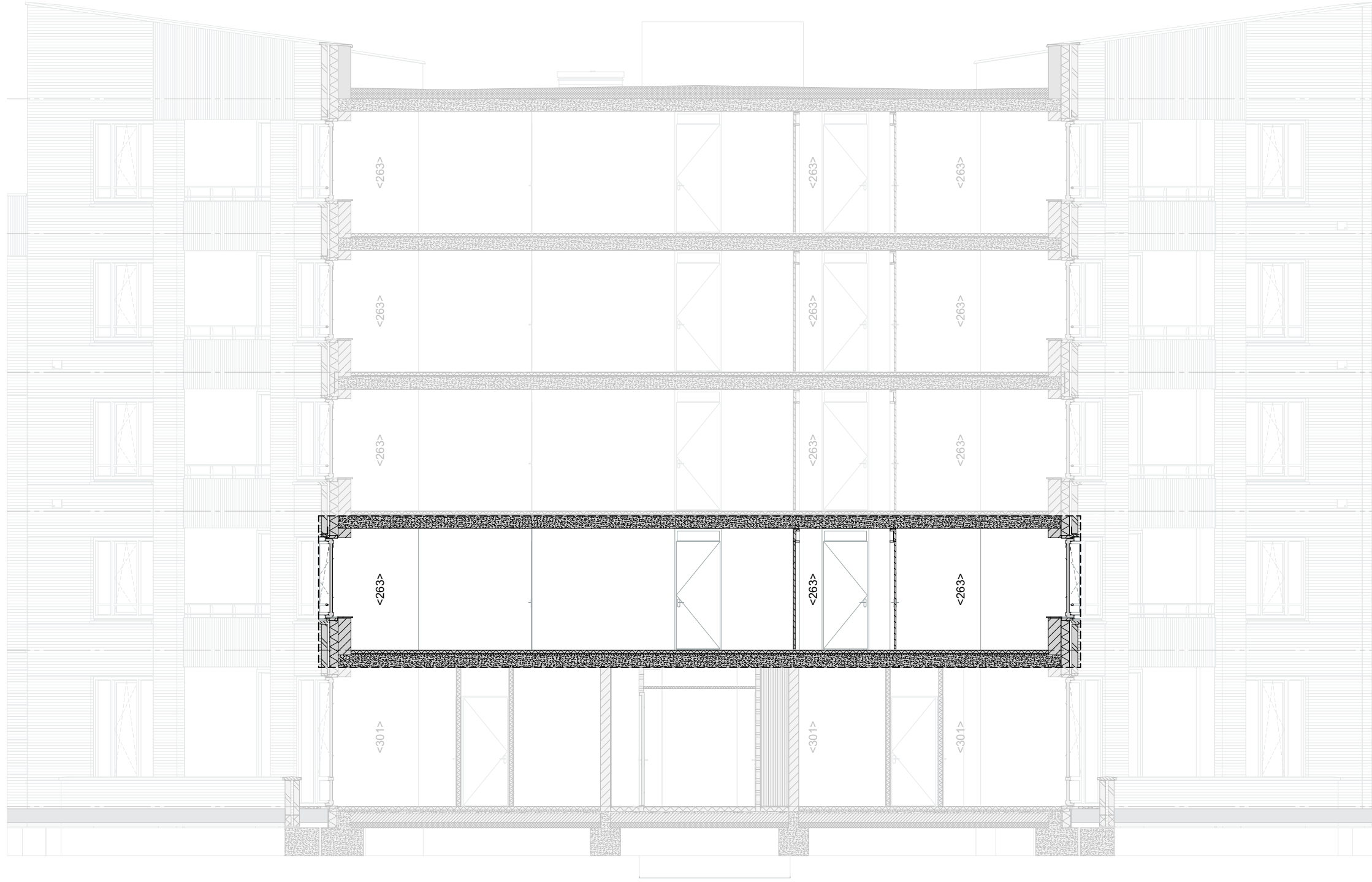
Doorsnede BB | 1:100
