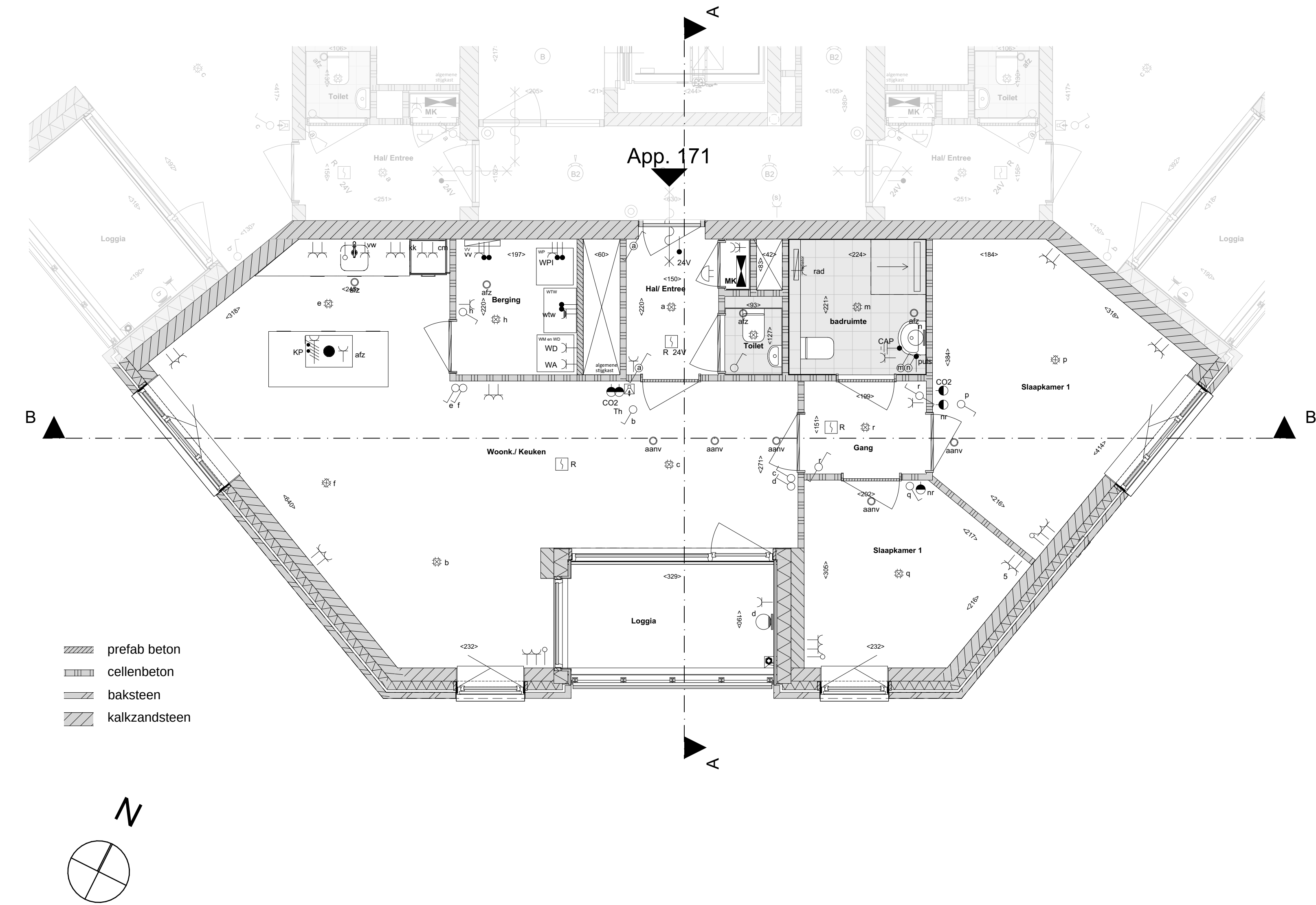
03 derde verdieping | 1:50
