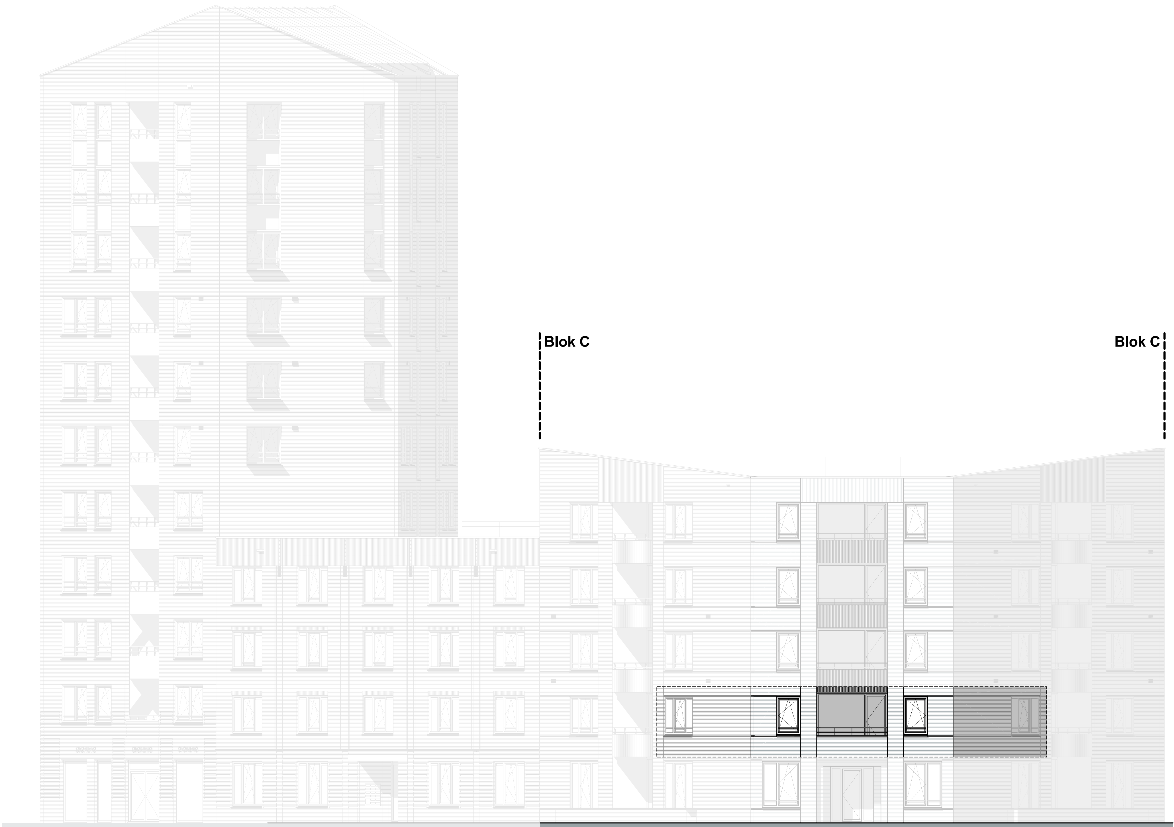
blok C G2 | 1:100
