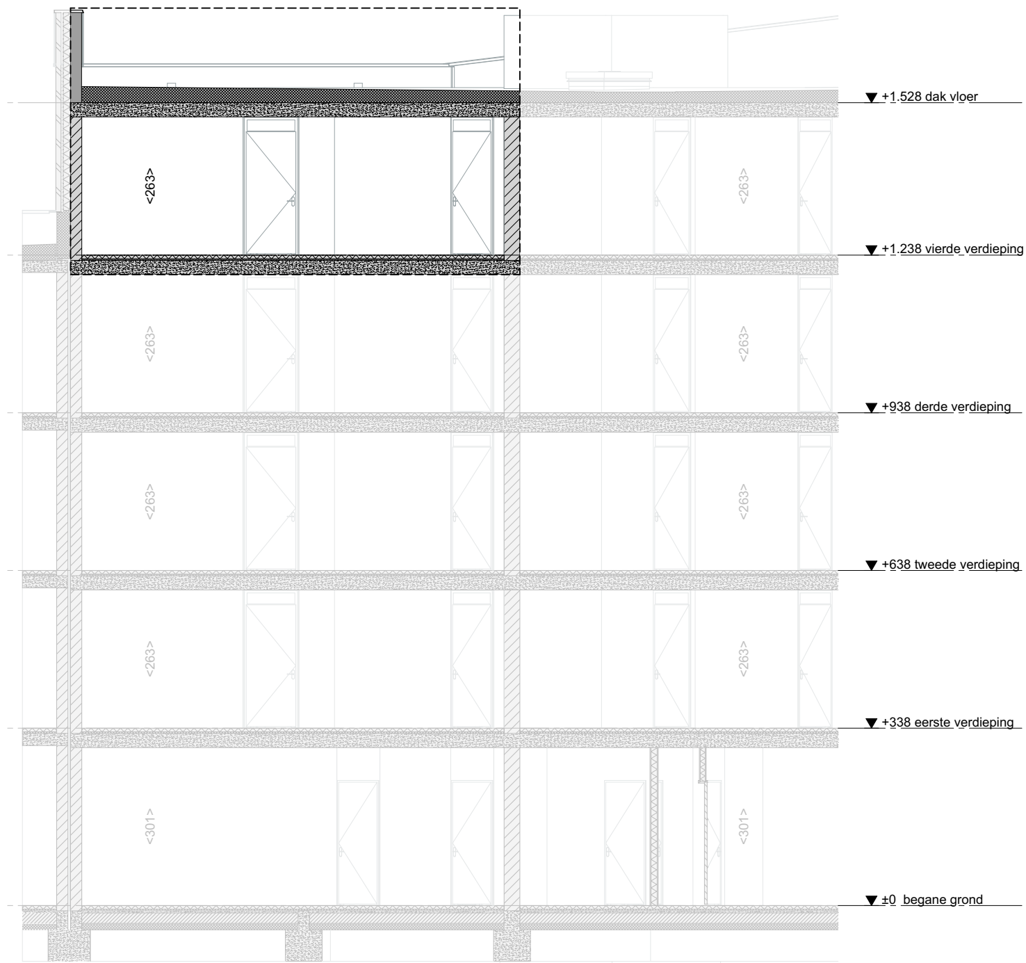
Doorsnede AA | 1:100
