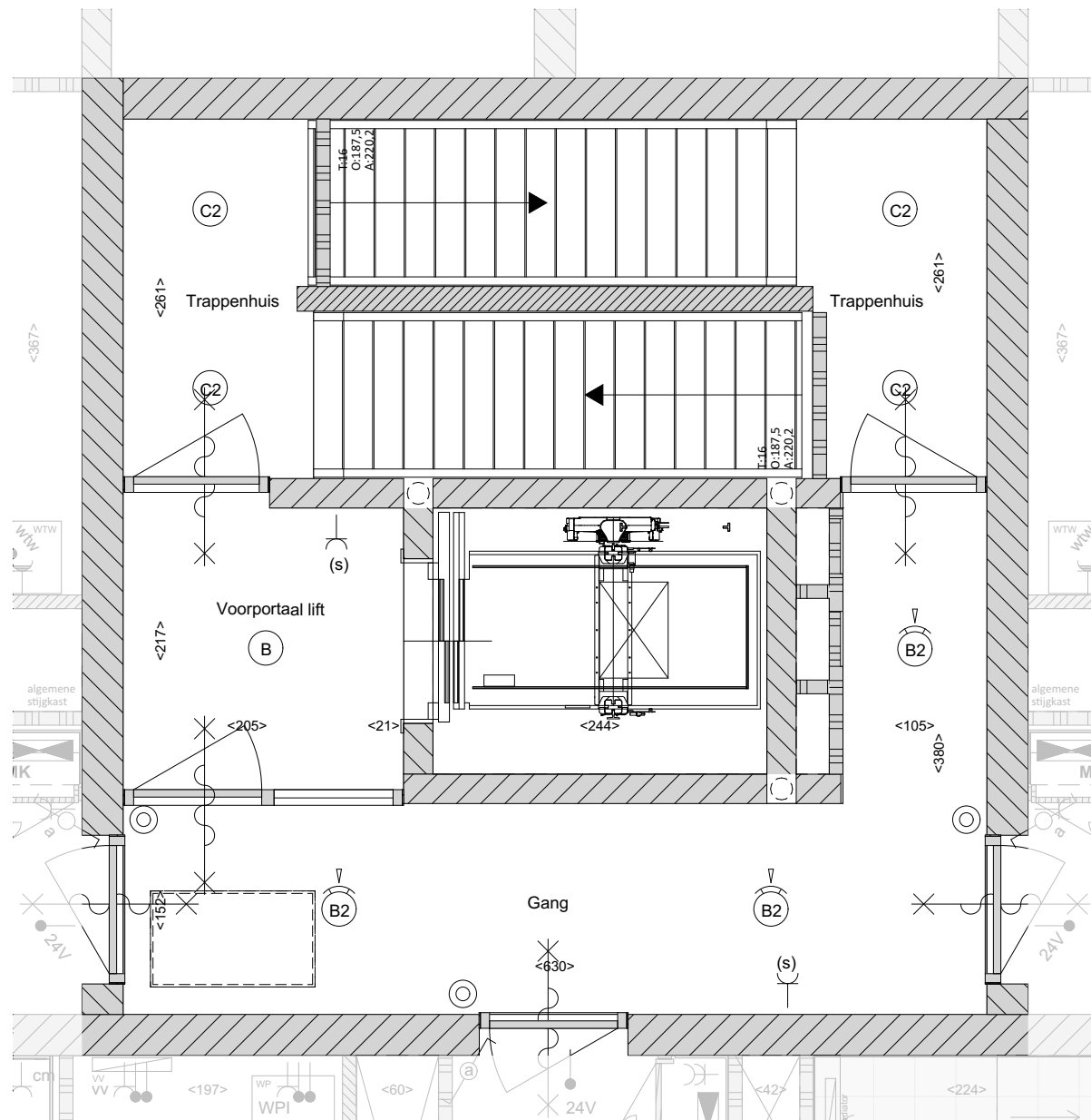
04 vierde verdieping | 1:50
