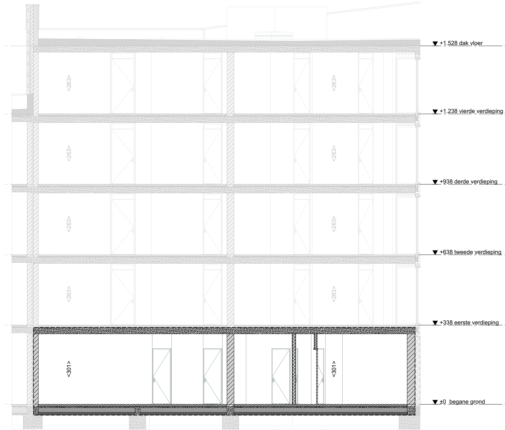
Doorsnede AA | 1:100
