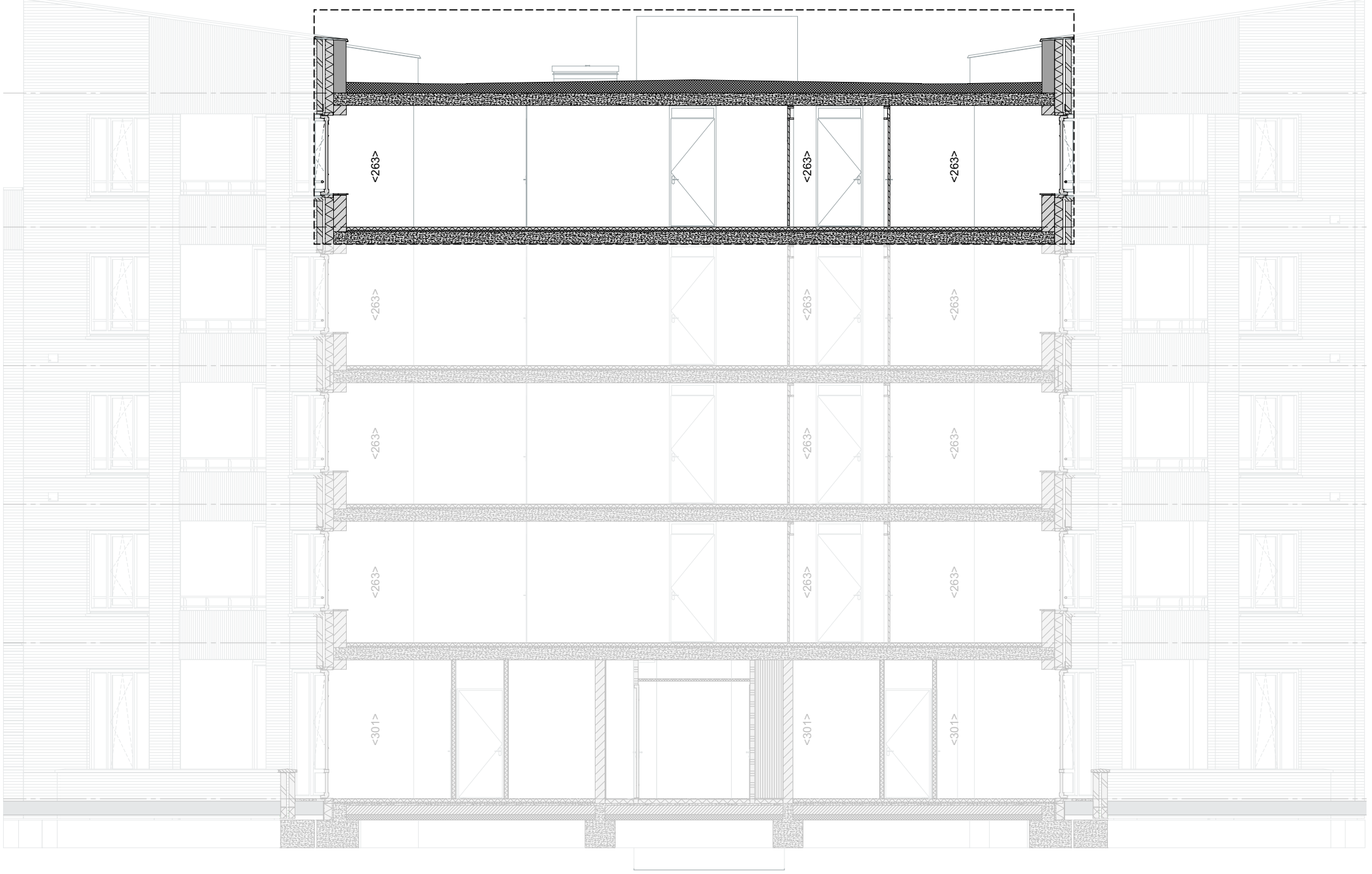
Doorsnede BB | 1:100
