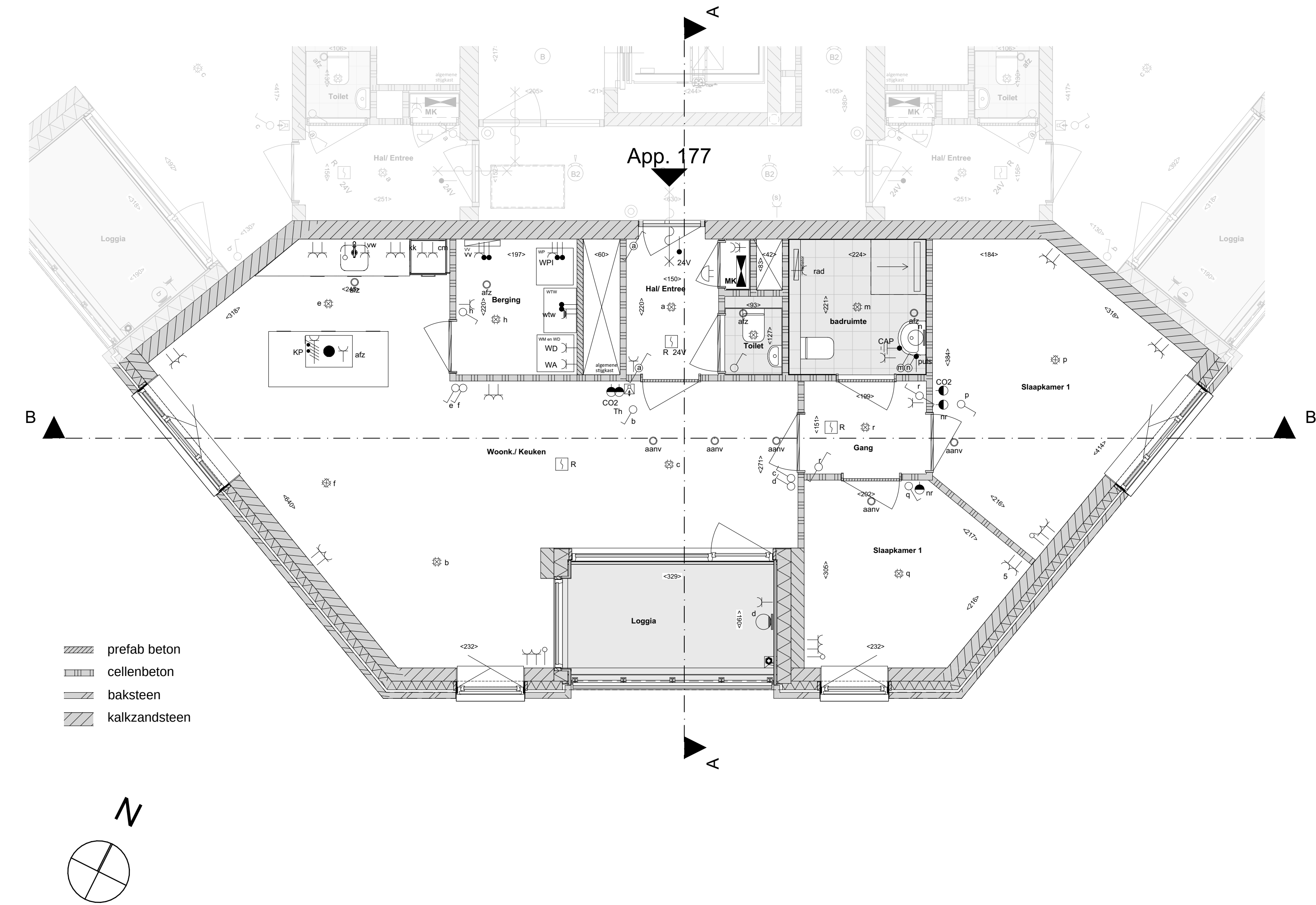
04 vierde verdieping | 1:50
