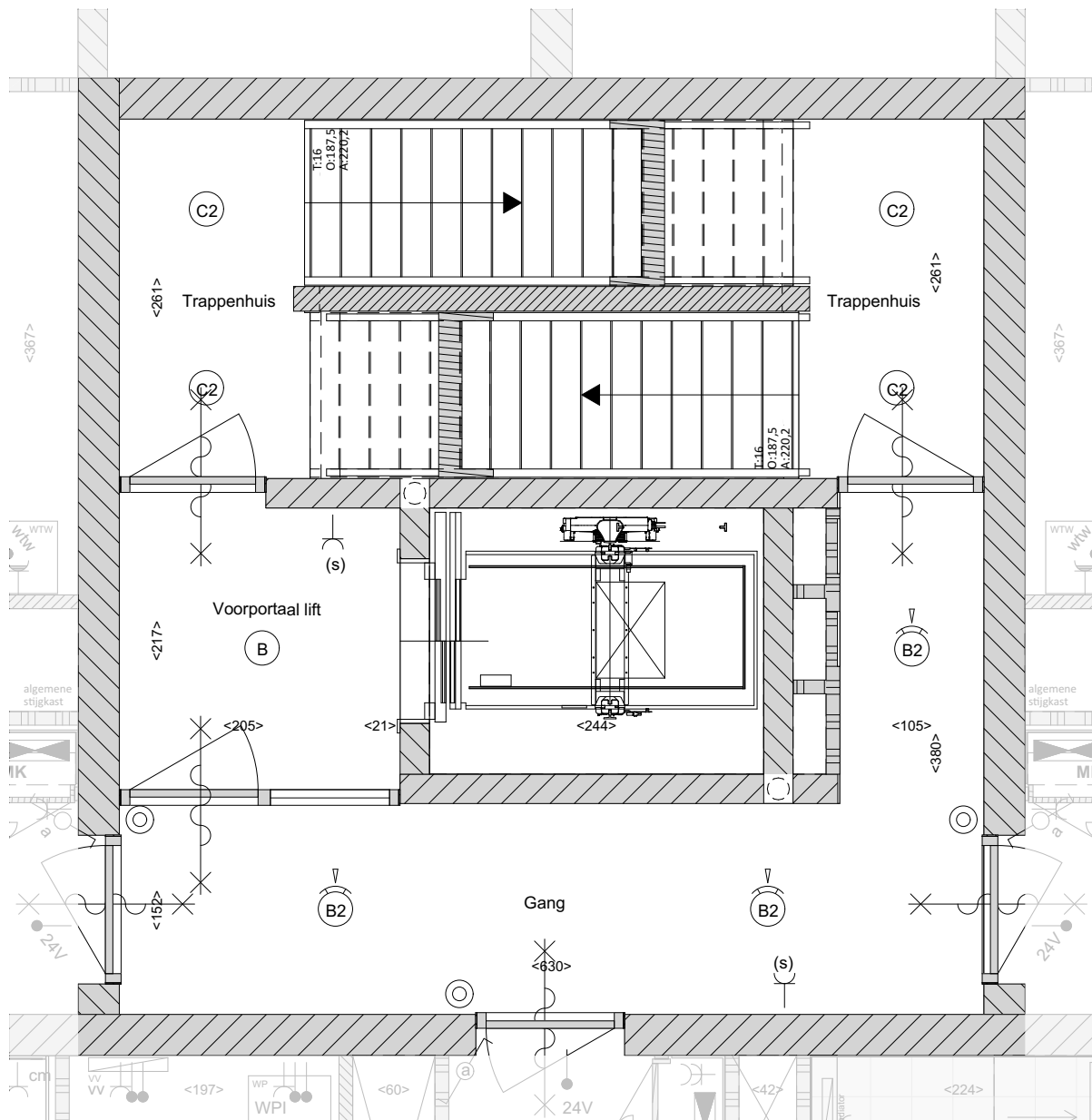
03 derde verdieping | 1:50
