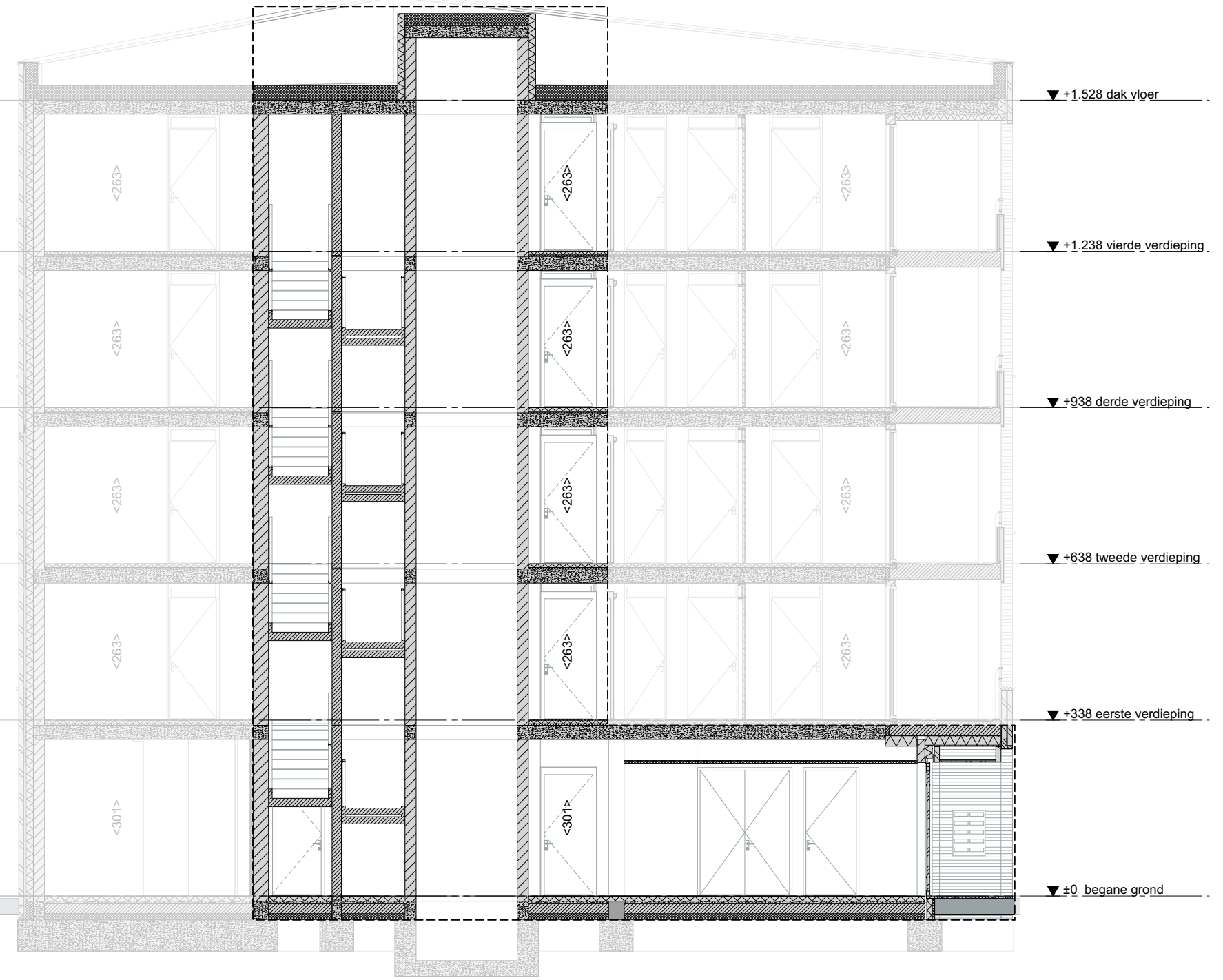
Doorsnede AA | 1:100
