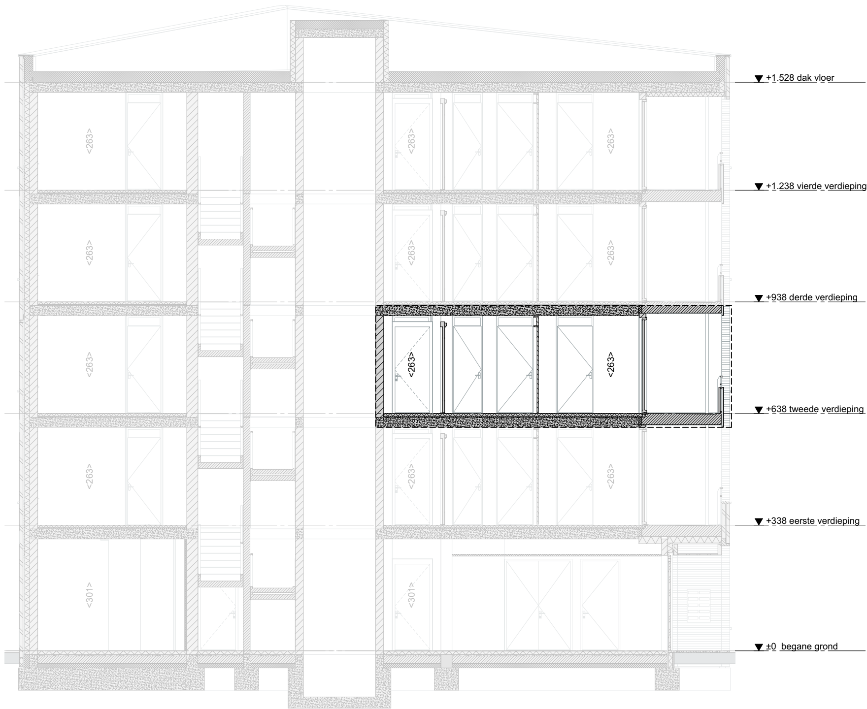
Doorsnede AA | 1:100
