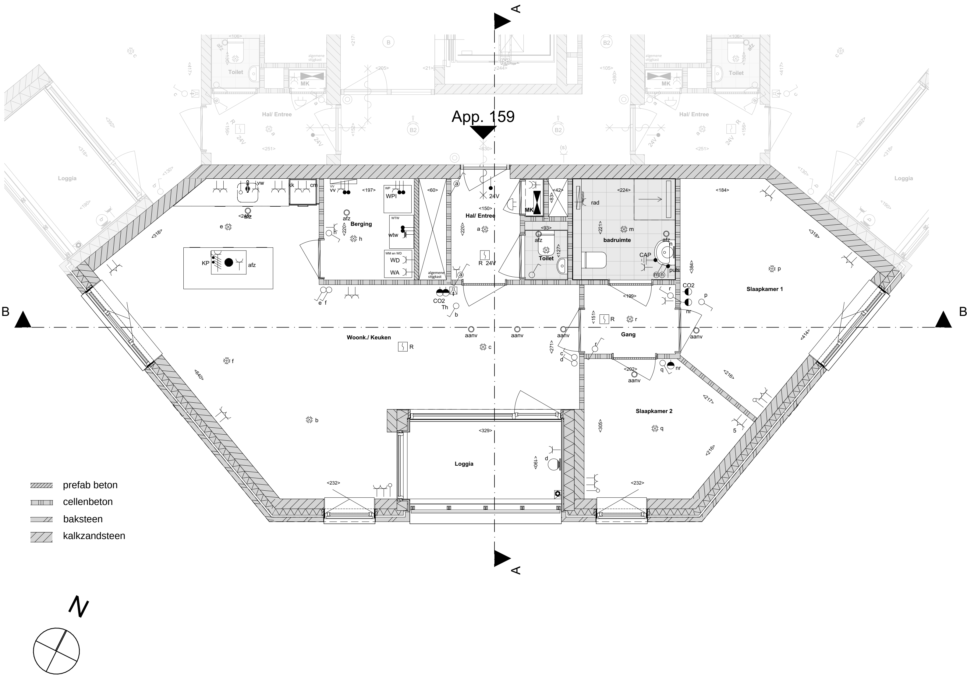
01 eerste verdieping | 1:50
