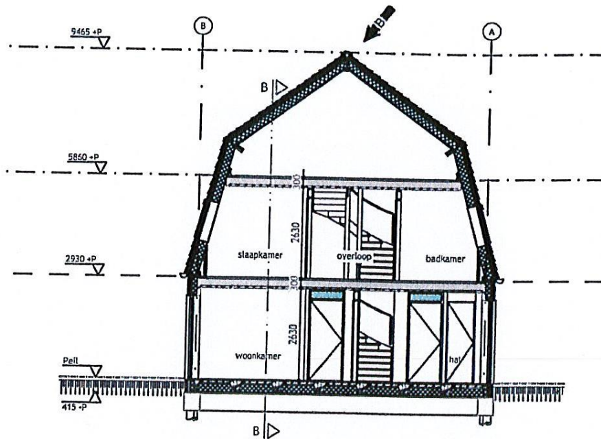
doorsnede A-A
