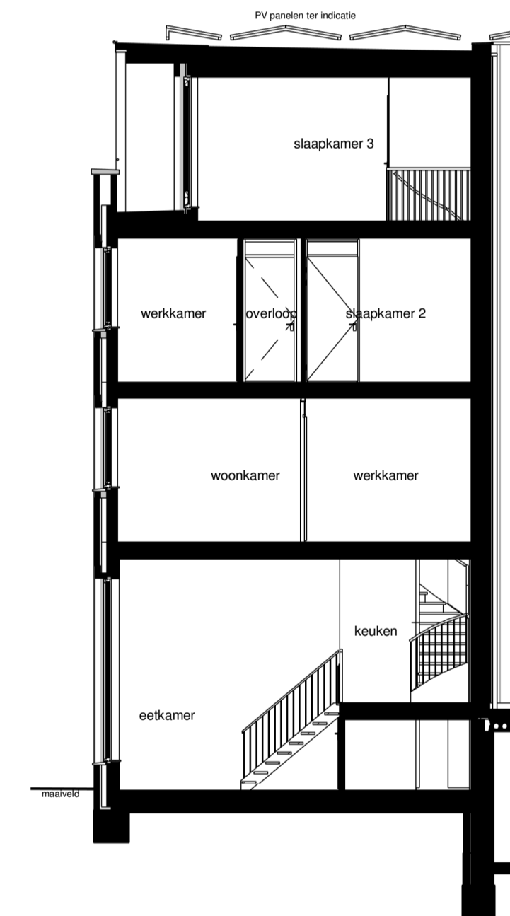
Doorsnede B schaal 1:100
