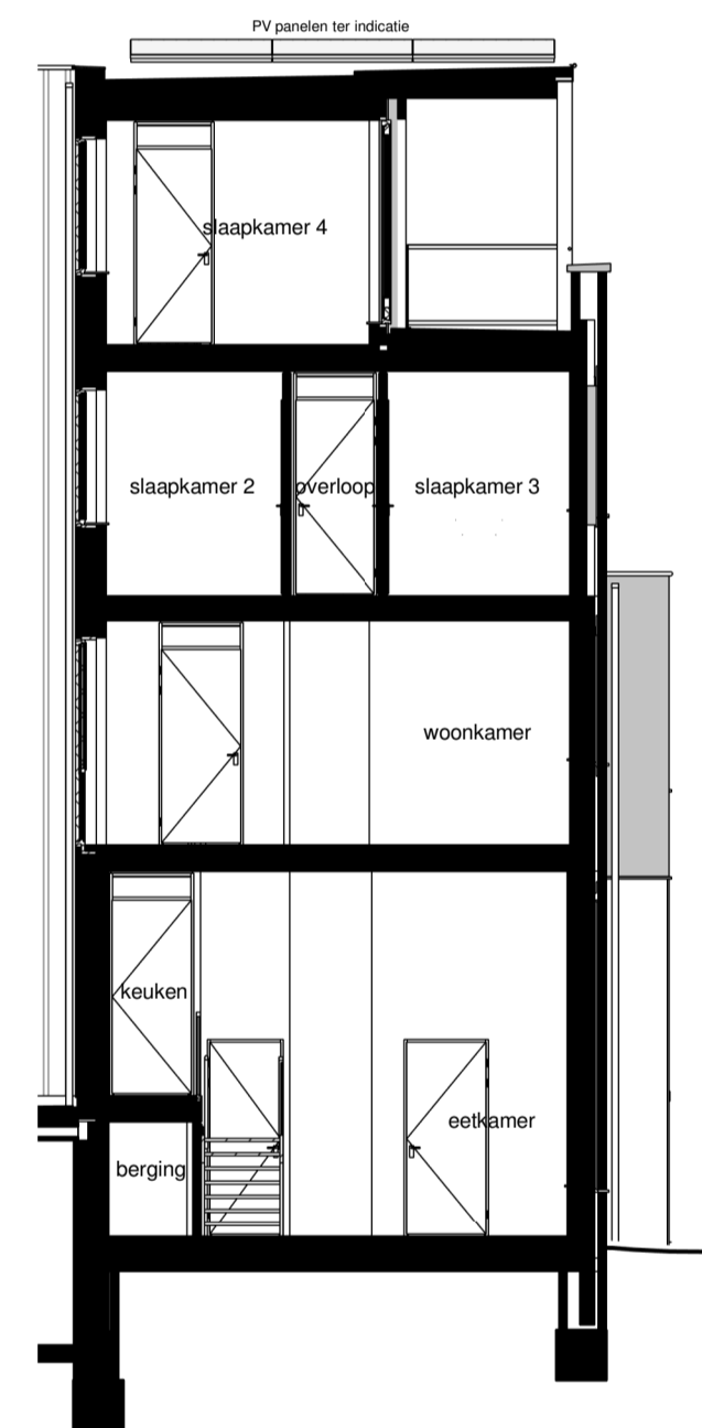
Doorsnede C schaal 1:100
