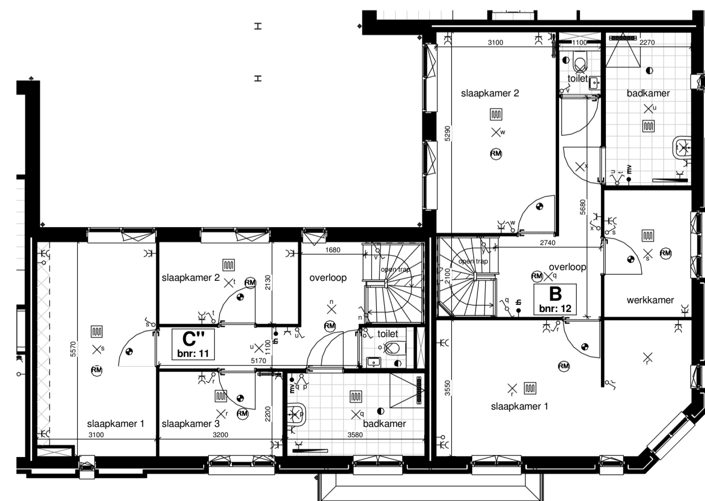
Derde verdieping schaal 1:100
