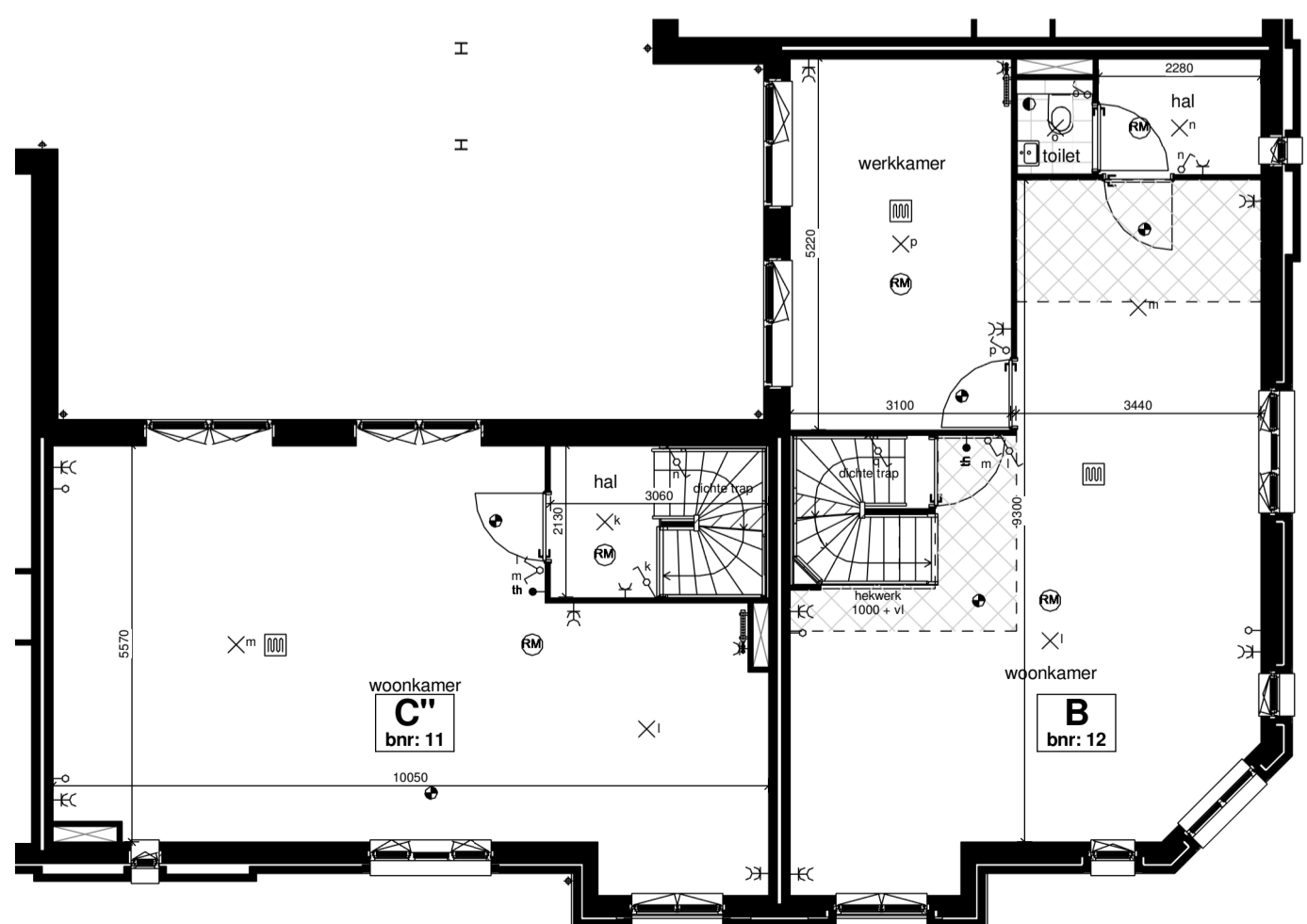
Tweede verdieping schaal 1:100
