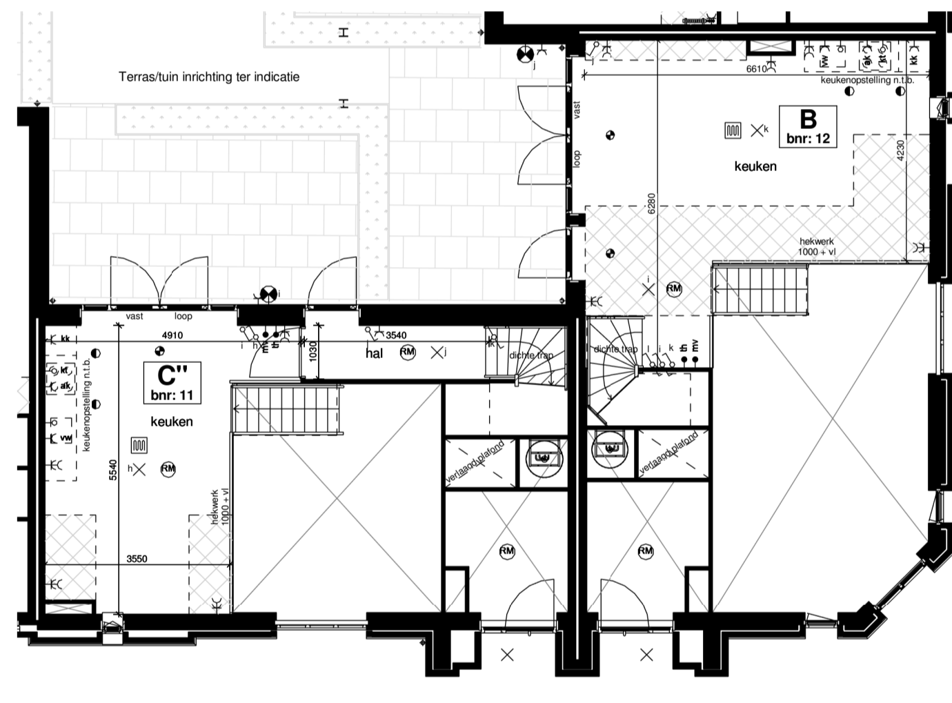
Eerste verdieping schaal 1:100
