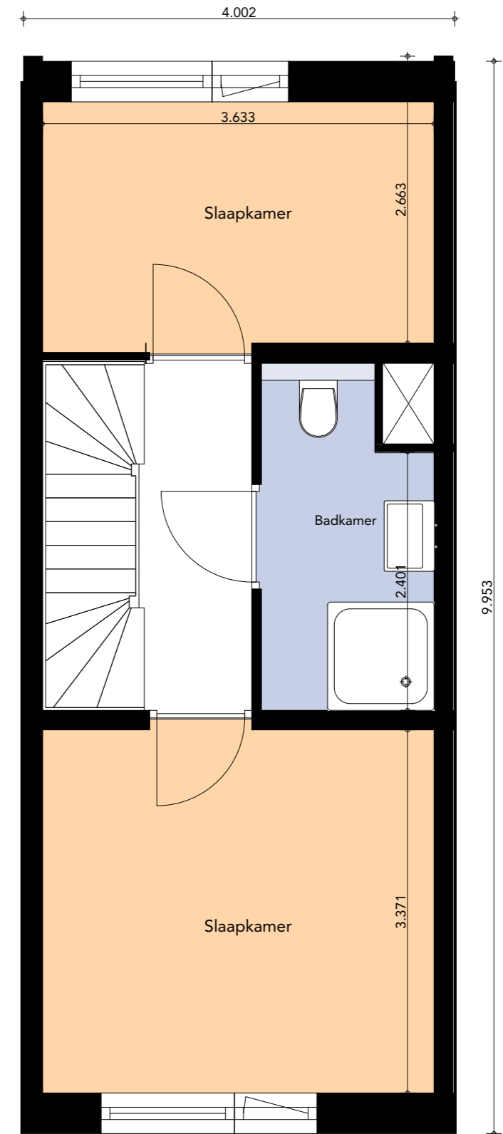
3e verdieping
