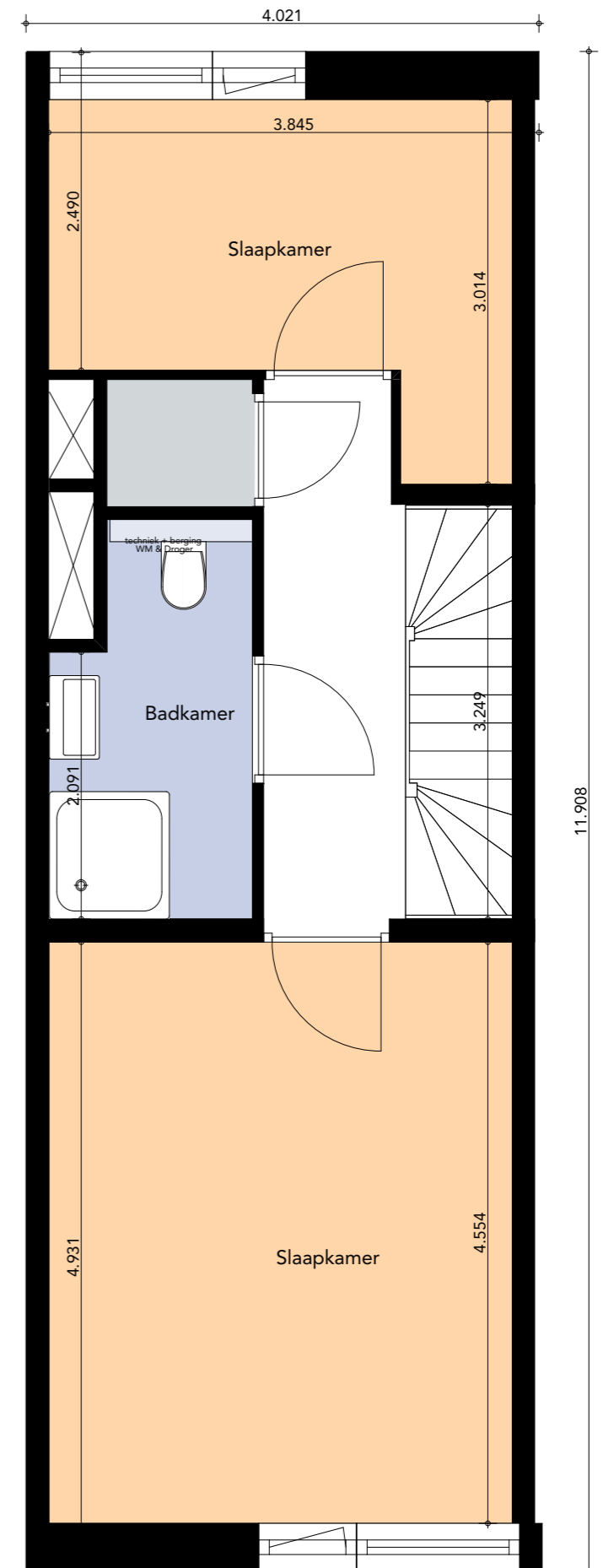
3e verdieping
